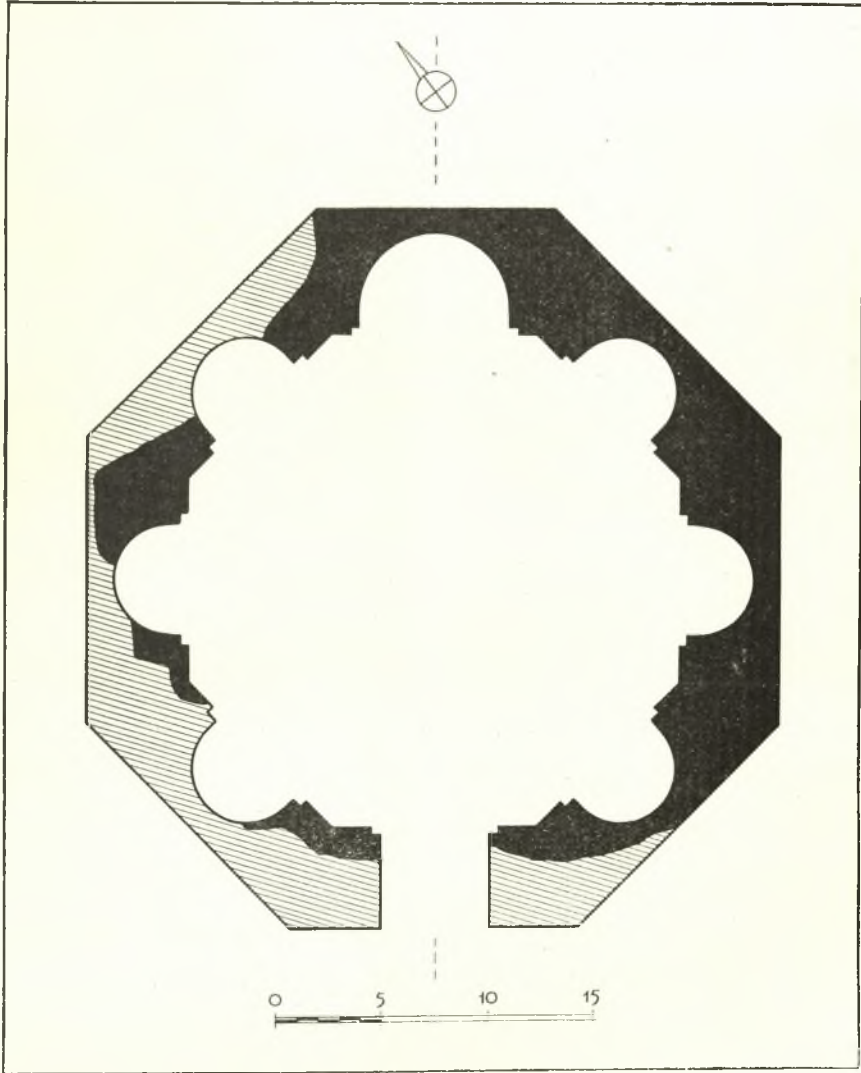
Εἰκ. 2. Κάτοπις τοῦ ὀκταγώνου συμπληρωμένη.
