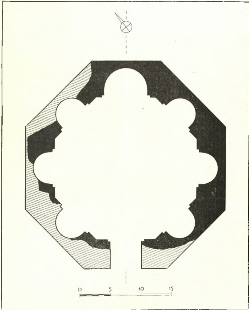
Εἰκ. 2. Κάτοπις τοῦ ὀκταγώνου συμπληρωμένη.
