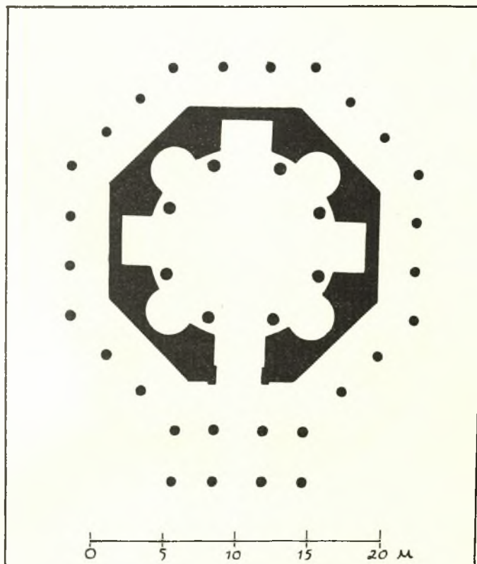
Εἰκ. 14. Κάτοπις τοῦ ἐν Σπαλάτῳ Μουσωλλείου τοῦ Διοκλητιανοῦ.
