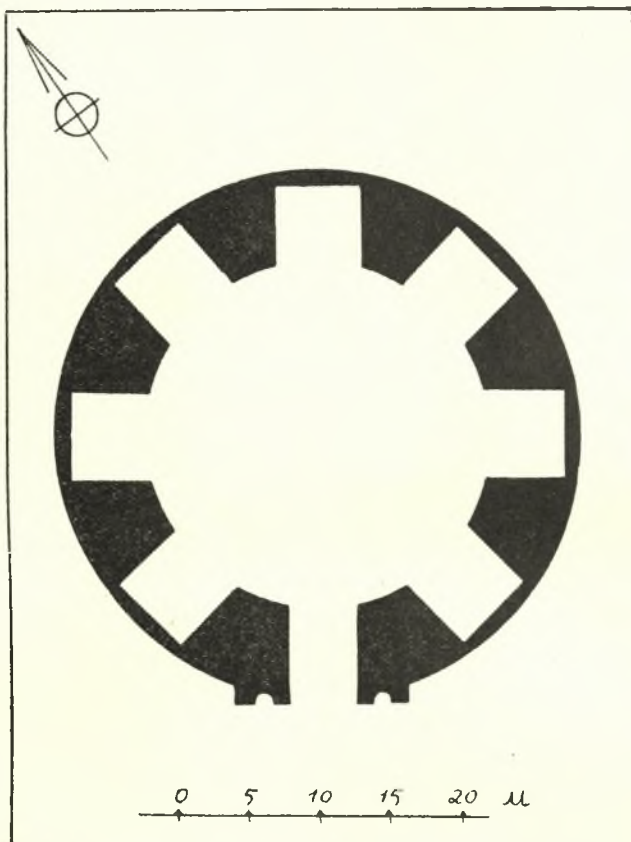
Εἰκ. 15. Κάτοψις τῆς ἐν Θεσσαλονίκῃ θόλου τοῦ Ἁγίου Γεωργίου.
