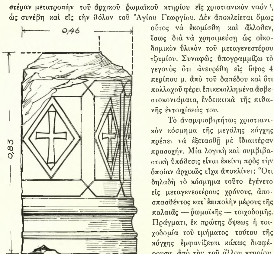
Εἰκ. 12. Πλαγία ὄψις τοῦ παλαιοχριστιανικοῦ ἄμβωνος.
