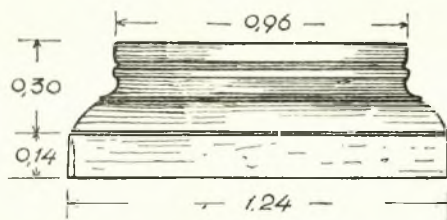
Εἰκ. 9. Βάσις κίονος.
