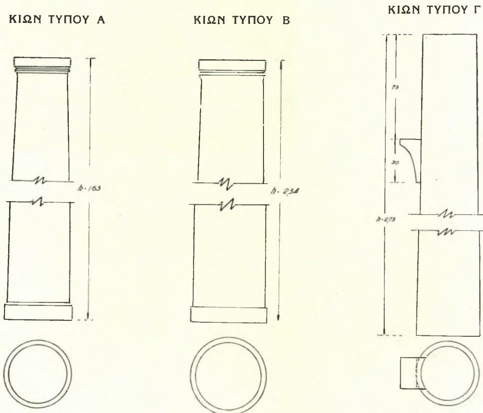
Εἰκ. 24. Κίων μετὰ συμφοῦς προβόλου.
