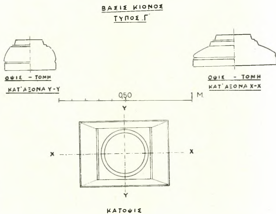
Εἰκ. 26. Βάσεις κίωνων τύπου Γ.
