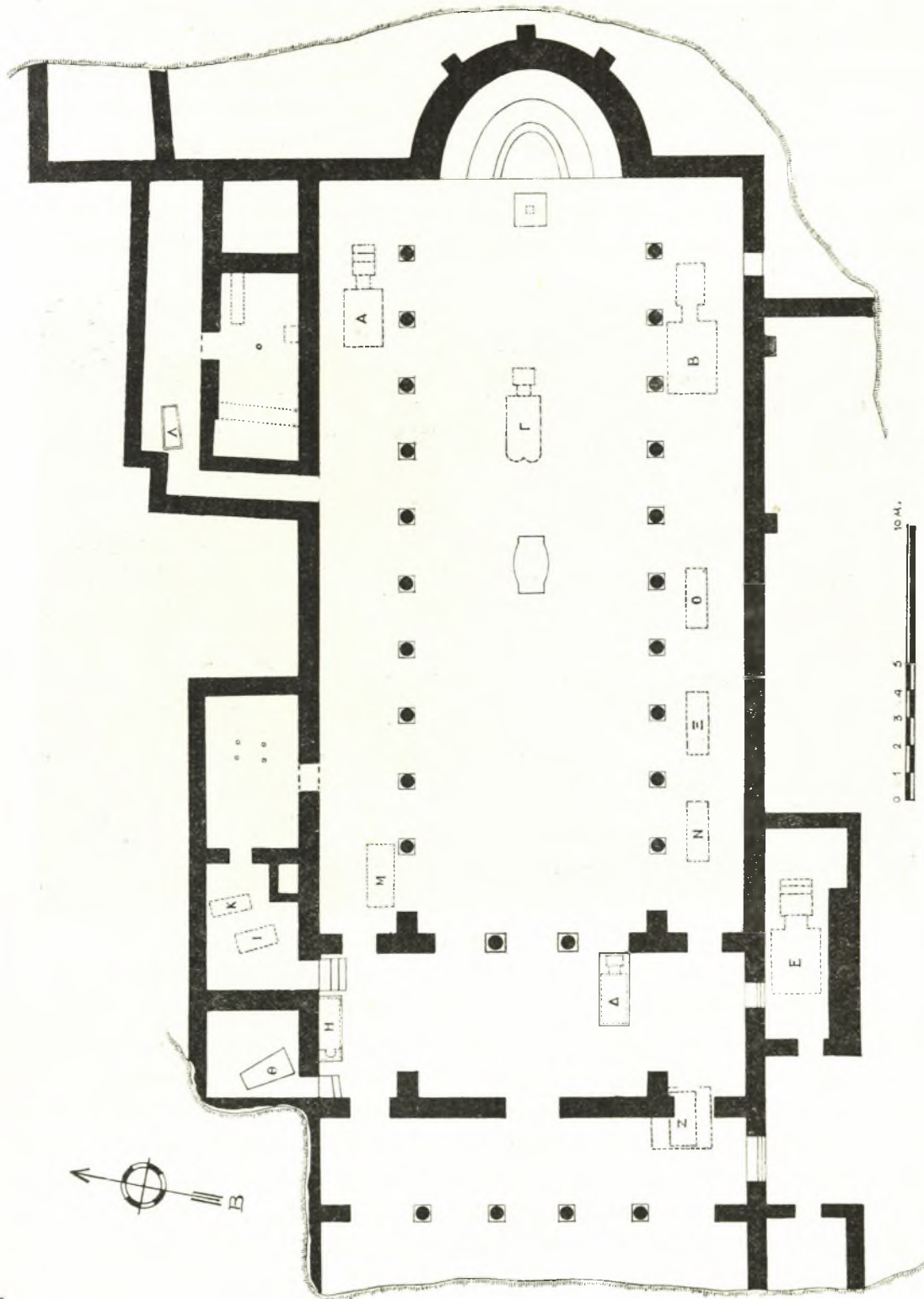
Εἰκ. 2. Ἡ βασιλικὴ τῶν Φιλίππων. Κάτοψις I (περίοδος α').
