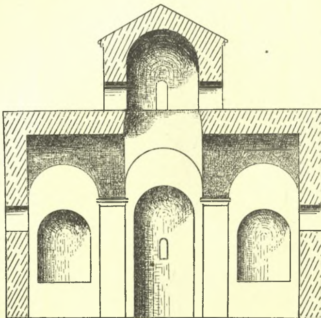
Εἰκ. 8. Ζεβρατίου ναοῦ τομὴ ἐγκαρσία.
