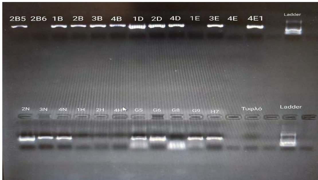
Εικόνα 14. Απεικόνιση αποτελεσμάτων PCR με universal COI primer, μέσω κάμερας UV.
