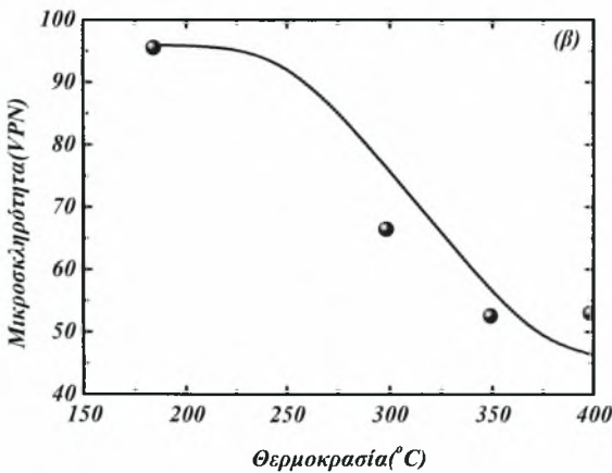
Σχήμα 3.4 : Σύγκριση πειραματικών τιμών και προβλέψεων του μοντέλου για επαναθέρμανση του κράματος 6 σε διάφορες θερμοκρασίες για 30 s. (α) Μεταβολή του αριθμού και του μέσου μεγέθους των σωματιδίων με την θερμοκρασία, (β) Μεταβολή της μικροσκληρότητας με την θερμοκρασία.
