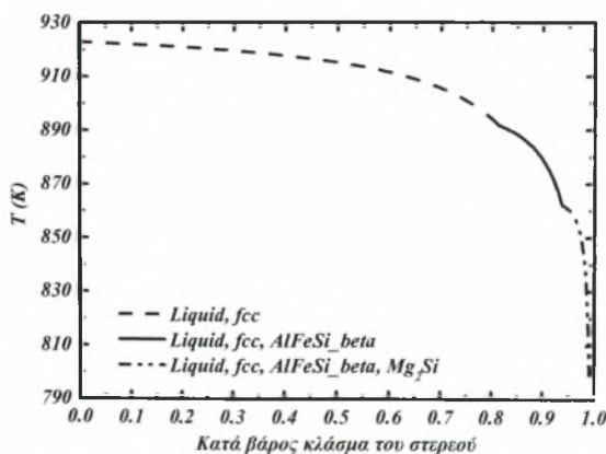
Σχήμα 4.3 : Πορεία Στερεοποίησης
