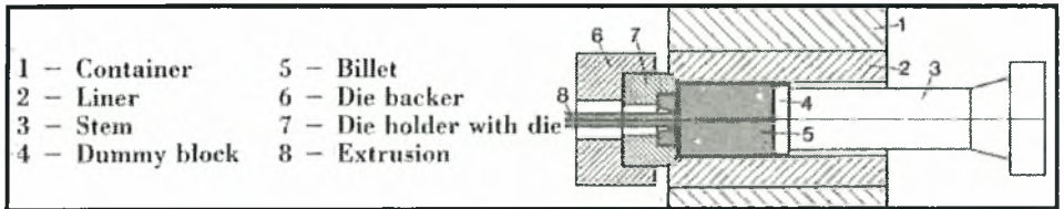
Σχήμα 1.1 : Σχηματικό διάγραμμα της διέλασης [1].
