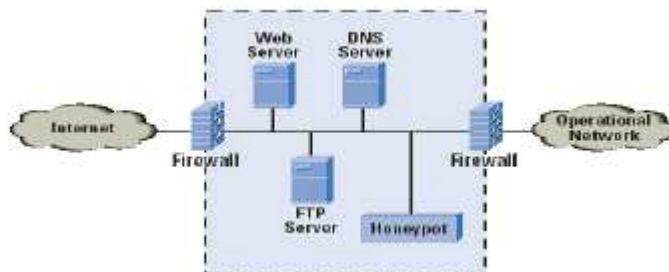
Εικόνα 4.6 : Υψηλής αλληλεπίδρασης honeybots.
