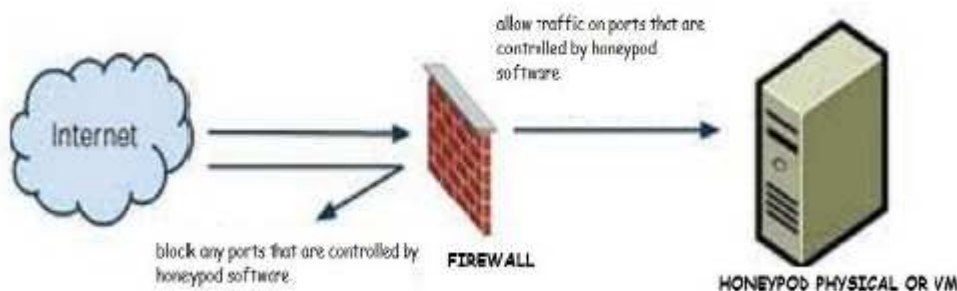
Εικόνα 4.5 : Χαμηλής αλληλεπίδρασης honeypots. Πηγή: Διπλωματική Εργασία Τσιρεπλή Ισμήνη "Honeyrots & Honeyd"
