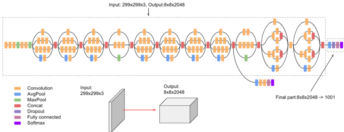
Εικόνα 5.7 – Αρχιτεκτονική Inception v3
