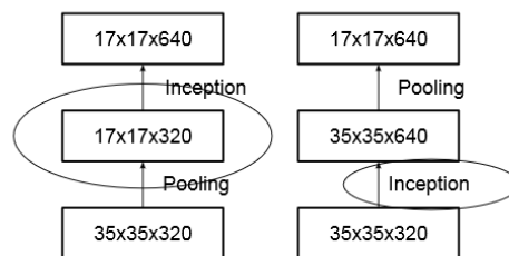
Εικόνα 5.6 – Reducing Grid Size
