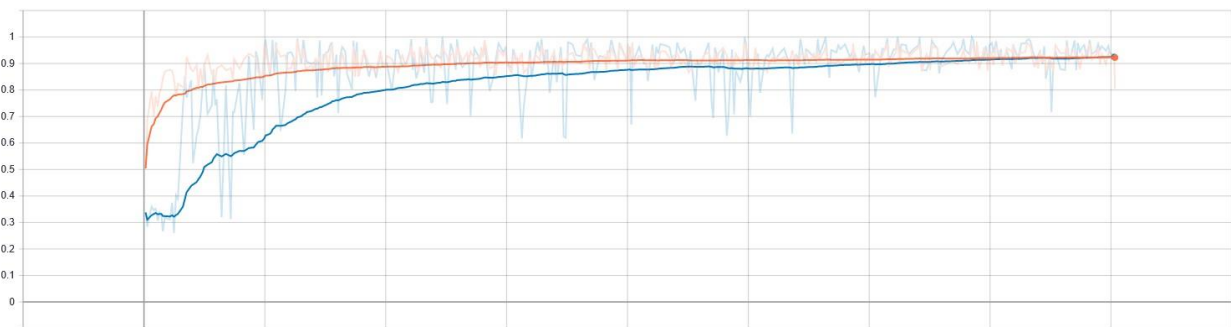
Εικόνα 5.9 – Validation (μπλε χρώμα)/Training (πορτοκαλί χρώμα) Accuracy μοντέλο Xception
