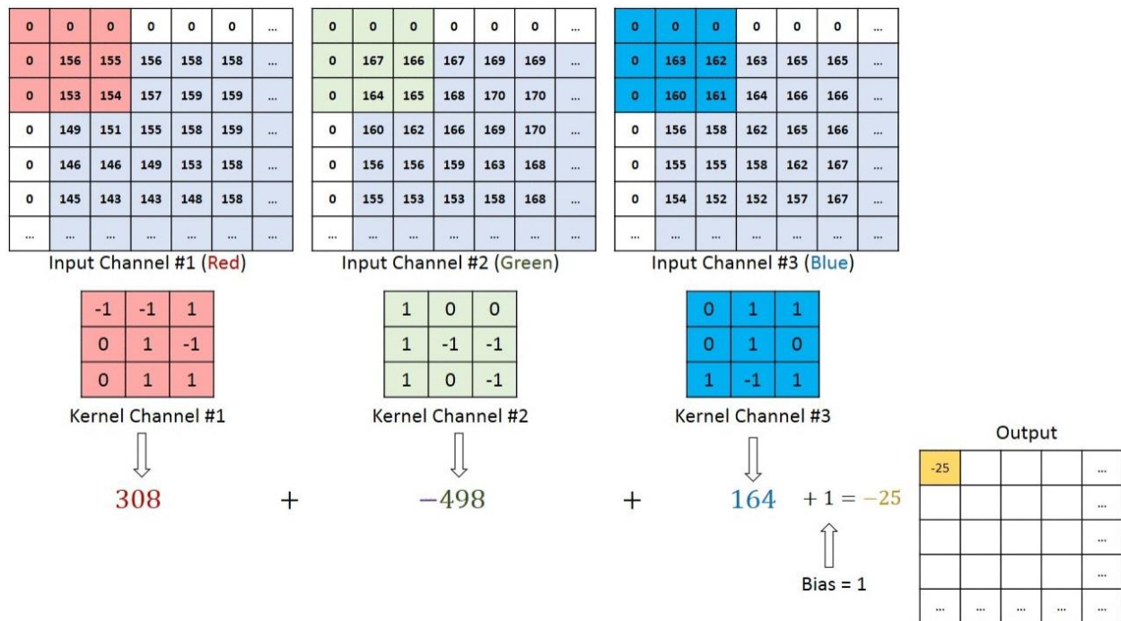
Εικόνα 3.15 – Διαδικασία Συνέλιξης Τριών Καναλιών
