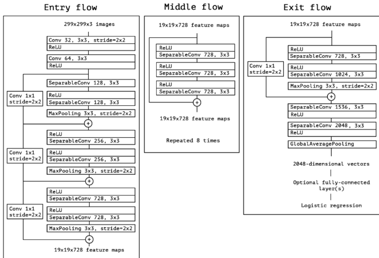
Εικόνα 5.8 – Αρχιτεκτονική Xception
