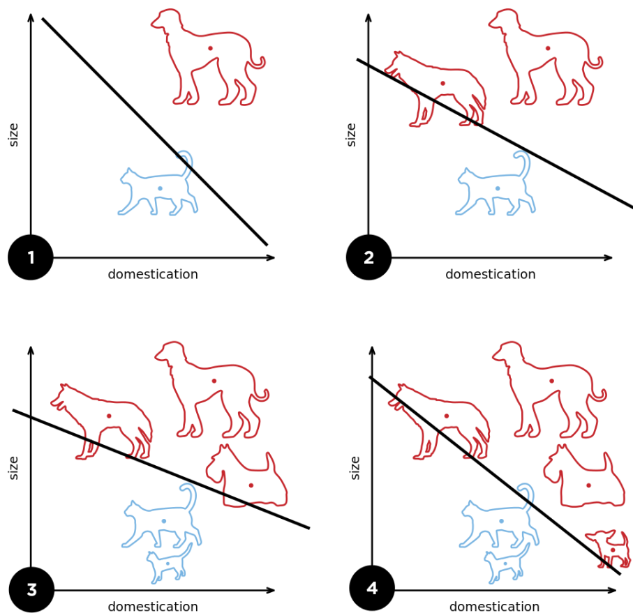
Εικόνα 3.3 – Στάδια κατηγοριοποίησης σύμφωνα με τον όγκο δεδομένων
