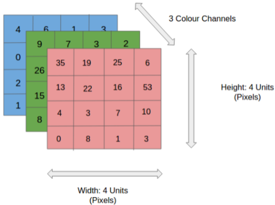
Εικόνα 3.13– Κανάλια Εικόνας (4x4x3)
