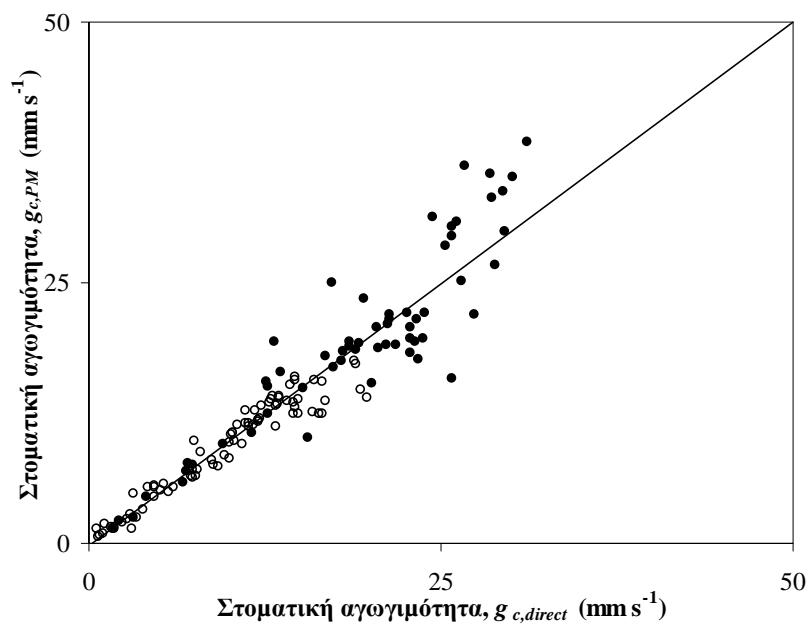
Σχήμα 6.8. Σύγκριση της στοματικής αγωγιμότητας της καλλιέργειας, όπως υπολογίστηκε από την εξίσωση των Penman-Monteith g_{c,PM} ( mm s^{-1} ), με τη στοματική αγωγιμότητα της καλλιέργειας, όπως υπολογίστηκε από την σχέση (2.29) g_{c,direct} ( mm s^{-1} ). (ο) 19-20-21 Αυγούστου, χωρίς δροσισμό, (●) 25-26-27 Αυγούστου, με δροσισμό.
