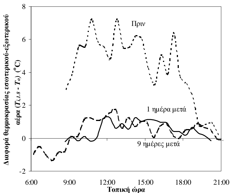
Σχήμα 5.2. Ημερήσια πορεία της διαφοράς θερμοκρασίας εσωτερικού-εξωτερικού αέρα \Delta T_{i-o} (= T_{i,1.8} - T_o) ( ^{\circ}\text{C} ), πριν το άσπρισμα, 28 Ιουνίου 1999 (- - -), αμέσως μετά, 8 Ιουλίου 1999 (—) και 9 ημέρες μετά, 16 Ιουλίου 1999 (— — —).
