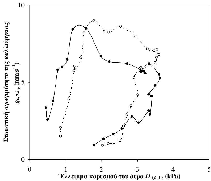
Σχήμα 4.9. (α) Στοματική αγωγιμότητα της καλλιέργειας g_{c,0.3} (mm s -1 ) συναρτήσει της εισερχόμενης ηλιακής ακτινοβολίας G_a (W m -2 ). (●), 8 Αυγούστου, δυναμικός αερισμός, (○), 10 Αυγούστου, φυσικός αερισμός. (β) Στοματική αγωγιμότητα της καλλιέργειας g_{c,0.3} (mm s -1 ) συναρτήσει του ελλείμματος κορεσμού του αέρα D_{i,0.3} (kPa). (●), 8 Αυγούστου, δυναμικός αερισμός, (○), 10 Αυγούστου, φυσικός αερισμός.
