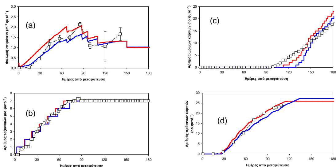
Σχήμα 8.4 (a), (b), (c), (d). Διακύμανση των μετρημένων ( \square ) και υπολογισμένων με το SimTom (—) & το BioSiGreT (—) μέσω τιμών της φυλλικής επιφάνειας, του αριθμού των ταξιανθιών, του αριθμού των ώριμων-συγκομιζόμενων και πράσινων-σηματιζόμενων καρπών, κατά τη διάρκεια της 1 ης πειραματικής περιόδου.
