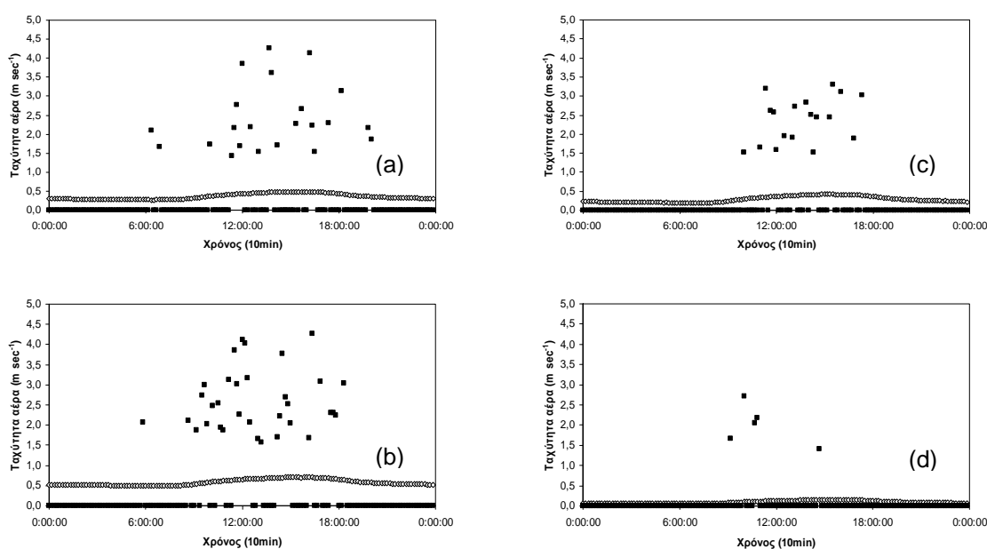
Σχήμα 9.11. Διακύμανση των μετρημένων ■ και υπολογισμένων ◇ τιμών της ταχύτητας του αέρα σύμφωνα με τη γεννήτρια κλιματικών δεδομένων για τις περιόδους: α). 1 Οκτωβρίου 2007, β). 5 Οκτωβρίου 2007, γ). 10 Φεβρουαρίου 2008, δ). 15 Μαρτίου 2008.
