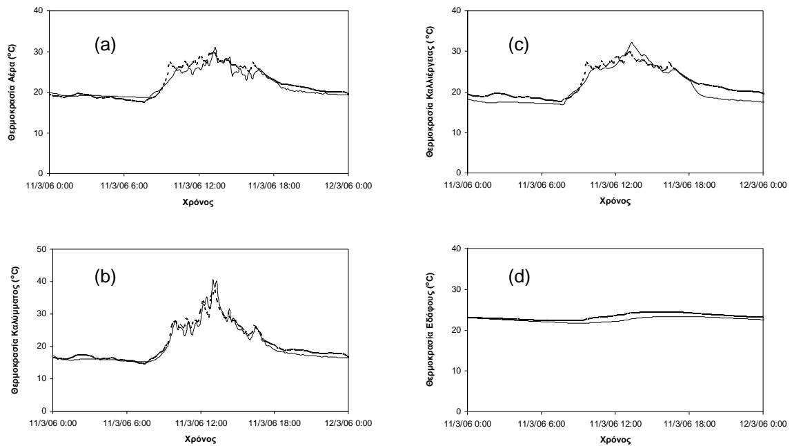
Σχήμα 8.1 (a), (b) (c), (d). Διακύμανση των μετρημένων (—) και υπολογισμένων (---) με χρήση του BioSiGreT τιμών, της θερμοκρασίας του αέρα, του καλύμματος της καλλιέργειας και του εδάφους, στις 11 Μαρτίου 2006.
