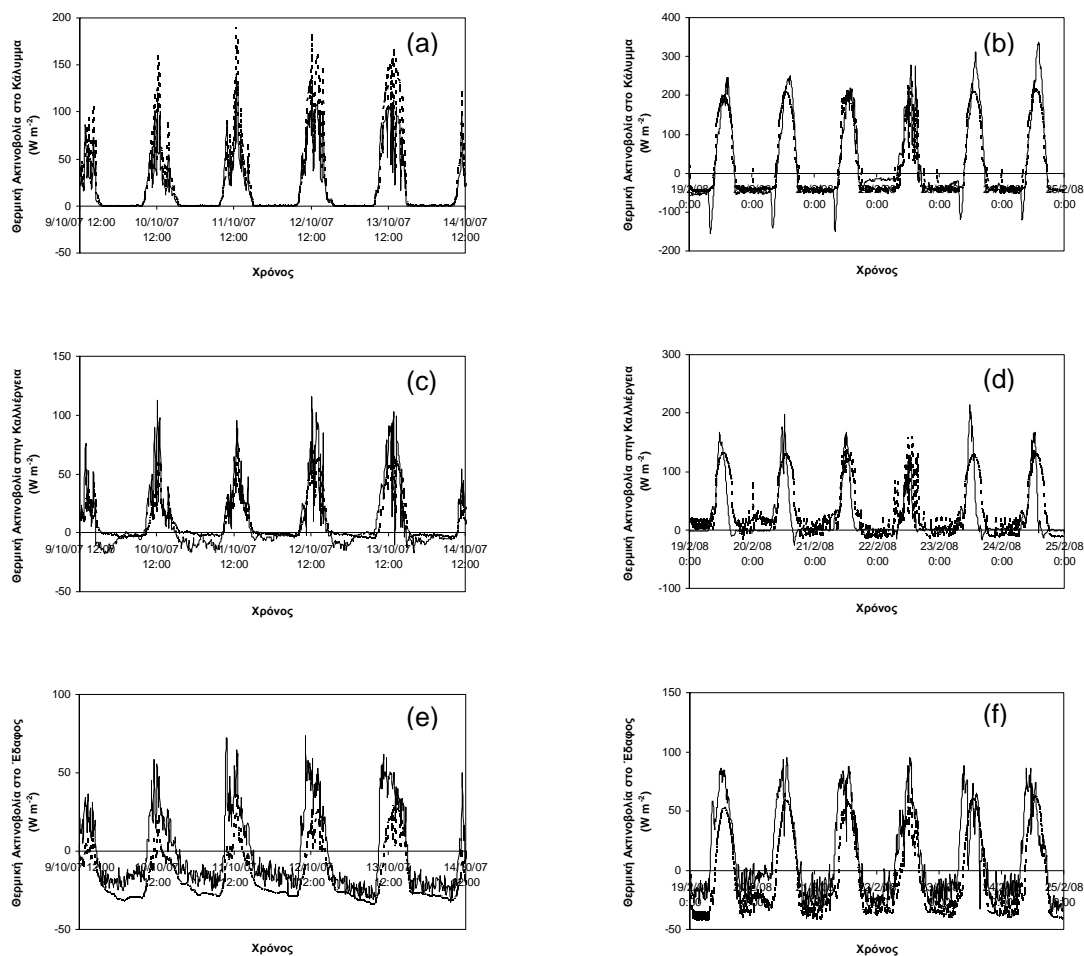
Σχήμα 6.11 (a), (b), (c), (d), (e), (f). Διακύμανση των μετρημένων (—) και υπολογισμένων (---) τιμών της καθαρής θερμικής ακτινοβολίας στο κάλυμμα, στην καλλιέργεια και στο έδαφος κατά τη διάρκεια δύο πειραματικών περιόδων.
