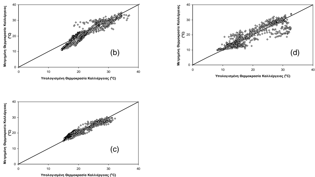
Σχήμα 6.8 (a), (b), (c), (d). Μετρημένες και υπολογισμένες τιμές της θερμοκρασίας της καλλιέργειας σε (1:1) απεικόνιση, για τις τρεις πειραματικές περιόδους.
