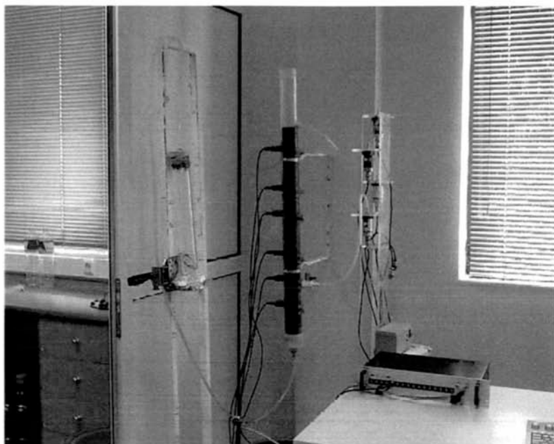
Εικόνα 4.4 Πειραματική διάταξη για τη μελέτη των χαρακτηριστικών καμπυλών του δεύτερου εδάφους [Αμμώδης Πηλός (SL)]
