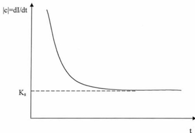
Σχήμα 2.5 Διηθητικότητα σε συνάρτηση με το χρόνο
