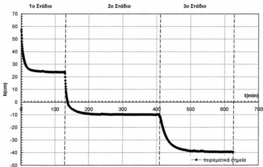
Σχήμα 4.35 Πίεση σε συνάρτηση με το χρόνο, κατά την 2 η στράγγιση [Αμμόδης Πηλός (SL)]
