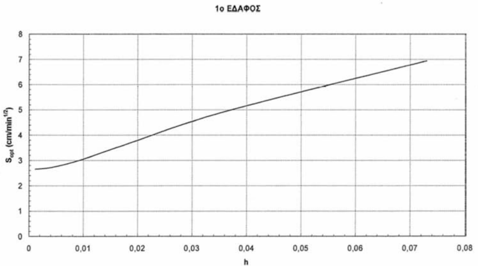
Σχήμα 5.8 Τιμές απορροφητικότητας αμμώδους εδάφους, που υπολογίστηκαν με τη μέθοδο 1/3 Simpson για διάφορα διαστήματα h
