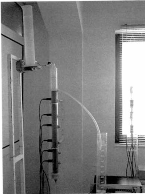
Εικόνα 4.2 Πειραματική διάταξη για τη μελέτη της αθροιστικής διήθησης
