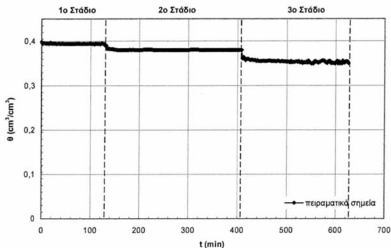
Σχήμα 4.34 Εδαφική υγρασία σε συνάρτηση με το χρόνο, κατά την 2 η στράγγιση [Αμμόδης Πηλός (SL)]
