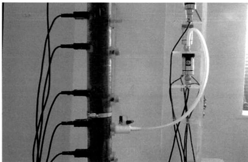
Εικόνα 4.5 Πειραματική διάταξη για τη μελέτη των χαρακτηριστικών καμπυλών του δεύτερου εδάφους [Αμμώδης Πηλός (SL)]
