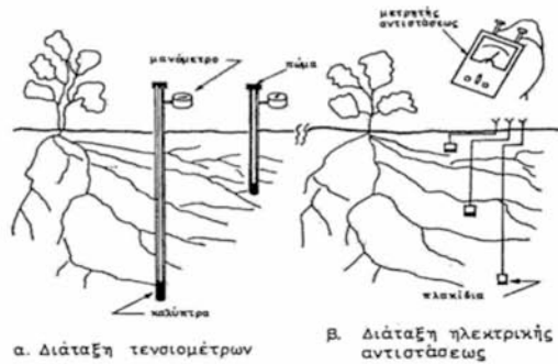
Σχήμα 3.1 Διάταξη тенσιομέτρων και πλακιδίων ηλεκτρικής αντίστασης για τον προσδιορισμό της τάσης της εδαφικής υγρασίας
