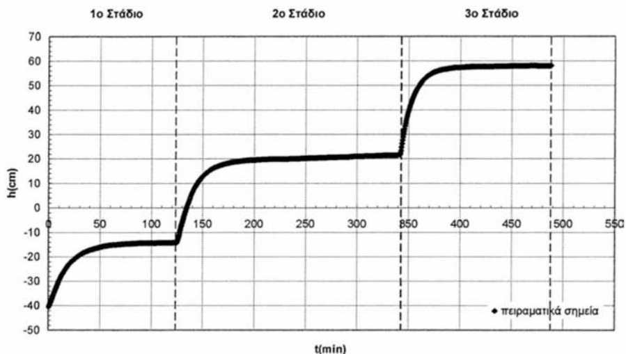
Σχήμα 4.33 Πίεση σε συνάρτηση με το χρόνο, κατά την 2 η διύγρανση [Αμώδης Πηλός (SL)]
