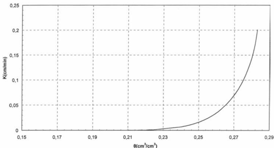
Σχήμα 5.23 Υδραυλική αγωγιμότητα σε συνάρτηση με την εδαφική υγρασία για την πηλώδη άμμο (RETc – αναλυτικό μοντέλο van Genuchten)
