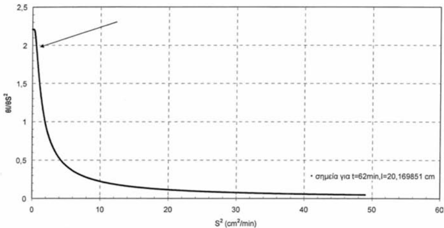
Σχήμα 5.25 Ανάλυση ευαισθησίας της παραμέτρου S^2 για μεγάλο χρόνο διάχυσης ( t = 62 min) [Πηλώδης Άμμος (LS)]
