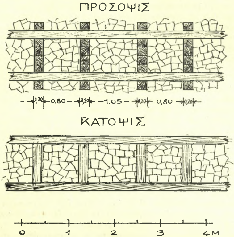
Εἰκ. 2. Πῶς φανταζόμεθα τὴν κτίσιν τοῦ βορείου τοίχου τοῦ αὐτοῦ δωματίου Ν (πρβλ. εἰκ. 1).
