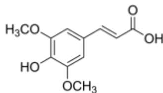
Συναπικό οξύ
