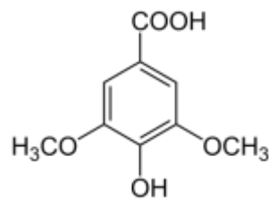
Συριγγικό οξύ
