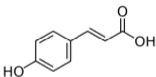
p-κουμαρικό οξύ
