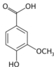
Βανιλλικό οξύ
