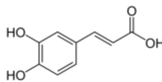
καφεϊκό οξύ
