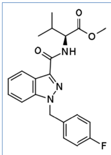
Εικόνα 21: Χημική δομή του AMB-FUBINACA ( https://commons.wikimedia.org )
