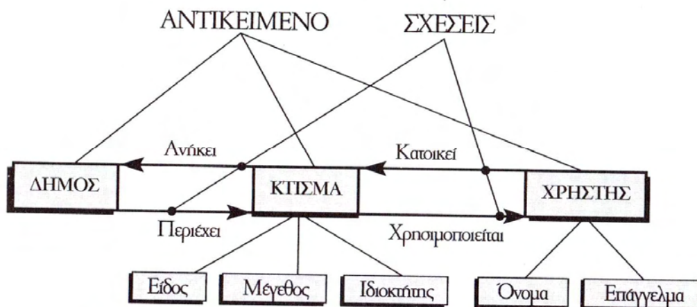
Σχήμα 1.4: Αντικειμενοστραφής Δομή
