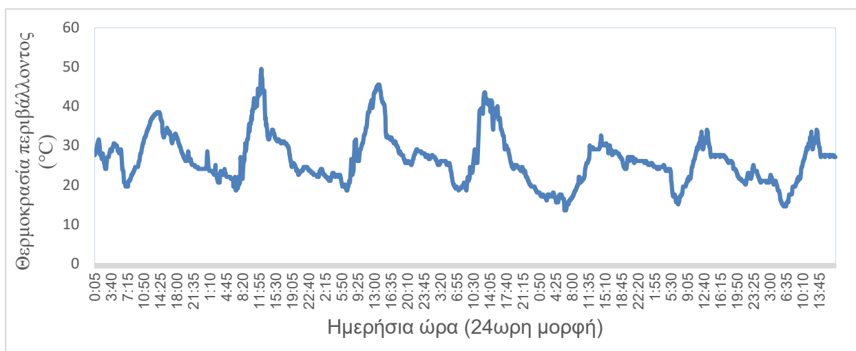
Εικόνα 24. Διακύμανση της θερμοκρασίας περιβάλλοντος κατά την διάρκεια της ημέρας στον MdS.
