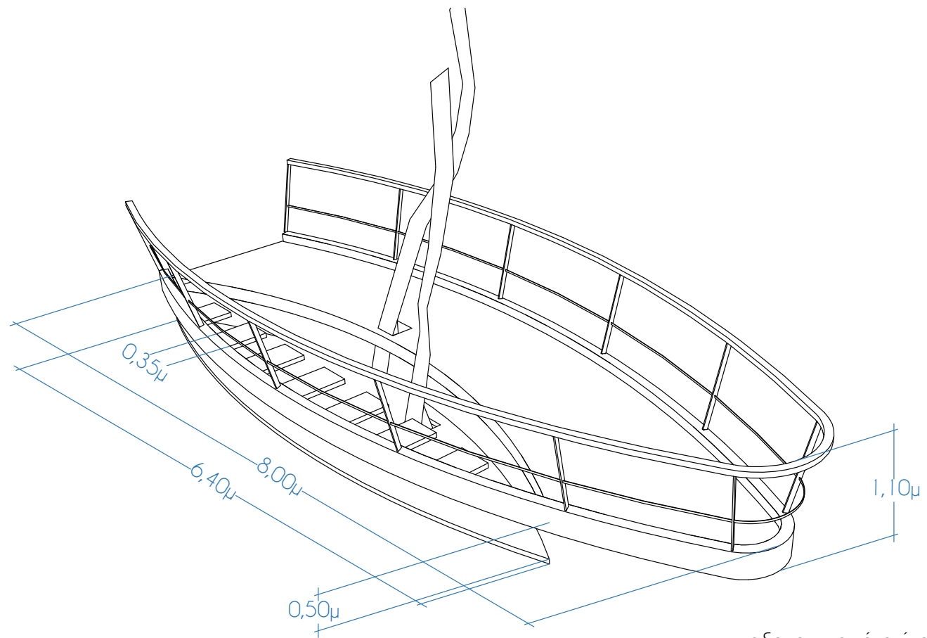
αξονομετρικό σκίτσο
