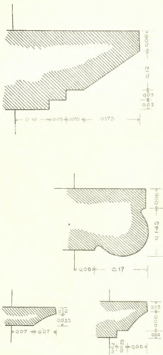
Εἰκ. 7. Γεῖσα. Ἄνω : πρώτου ὀρόφου. Μέσον : ἄνωθεν γυναικωνίτου. Κάτω ἄριστ. : δυτ. ἀνοίγματος, δεξ. βορ. καὶ νοτ. πλευρᾶς γυναικωνίτου.
