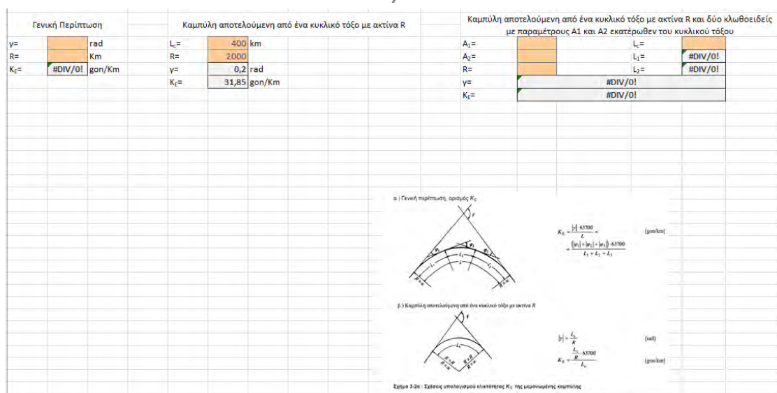
Εικόνα 11α: Υπολογισμός Ελικτούς K c (Κριτήριο Ασφ. I)
