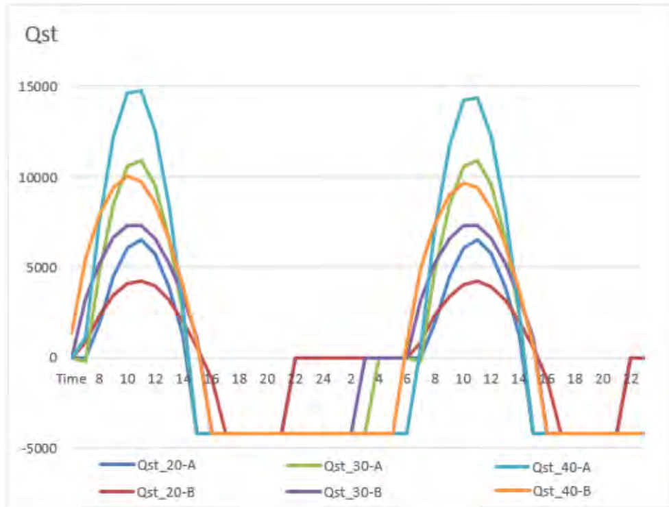
Σχήμα 4.6 Αποθηκευμένη ενέργεια στη δεξαμενή αποθήκευσης για περίοδο δύο ημερών για επιφάνεια 20,30,40 m 2 .
