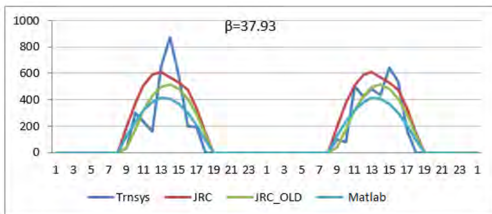
Σχήμα 4.23 Ακτινοβολία αλγορίθμου Matlab στην περιοχή της Αθήνας για την πρώτη ημέρα του Ιανουαρίου για γωνία \beta=\varphi σε σχέση με Trnsys και JRC.
