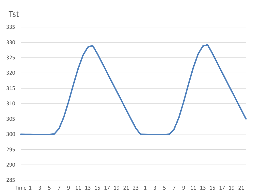
Σχήμα 4.33 Θερμοκρασία αποθήκευσης του φέροντος ρευστού για την τελευταία ημέρα του Οκτωβρίου και την πρώτη ημέρα του Νοεμβρίου.
