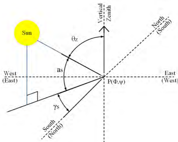
Εικόνα 2.6 Γωνίες συλλέκτη.
