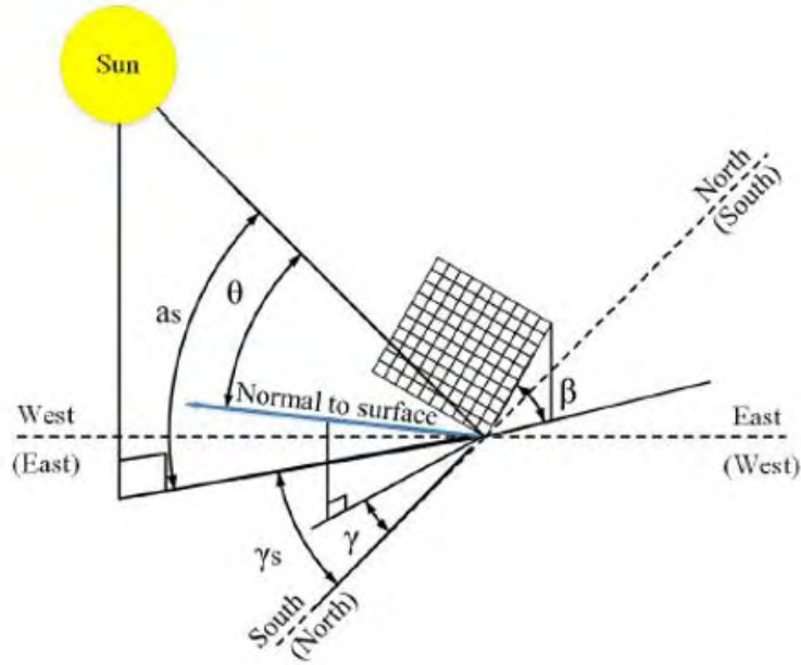
Εικόνα 2.5 Ηλιακές γωνίες.
