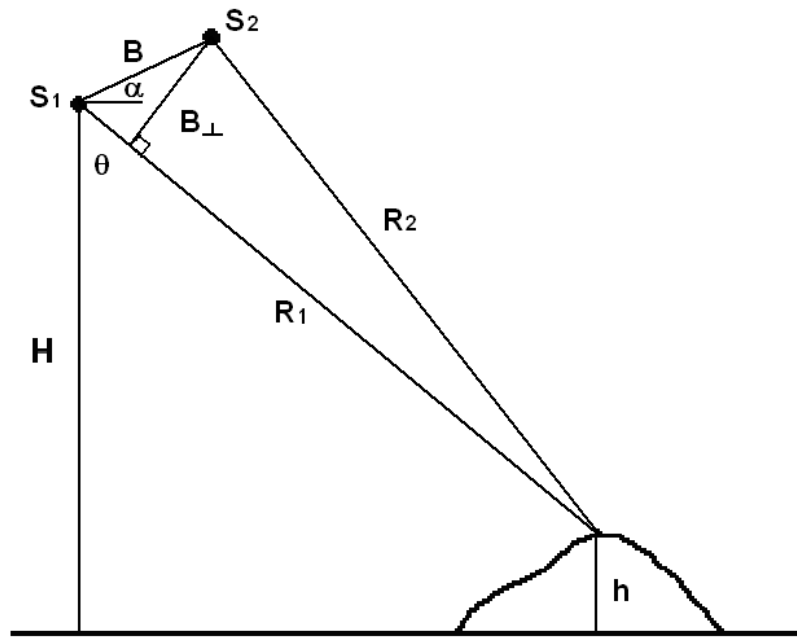
Εικόνα 3.4 Βασική γεωμετρία συμβολομετρικού συστήματος SAR (google)
