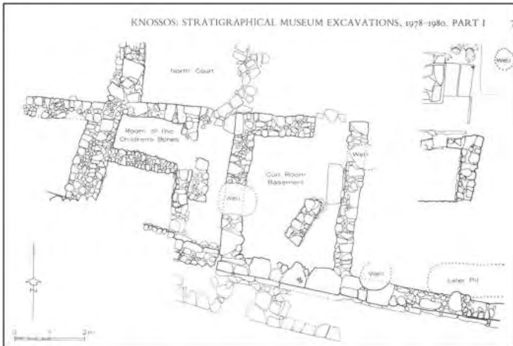
Εικόνα 5 Κάτοψη YM IB οίκου
