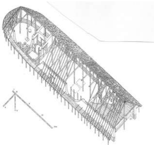
Εικόνα 23 Κάτοψη και Αναπαράσταση του Ηρώου, Λευκαντί
