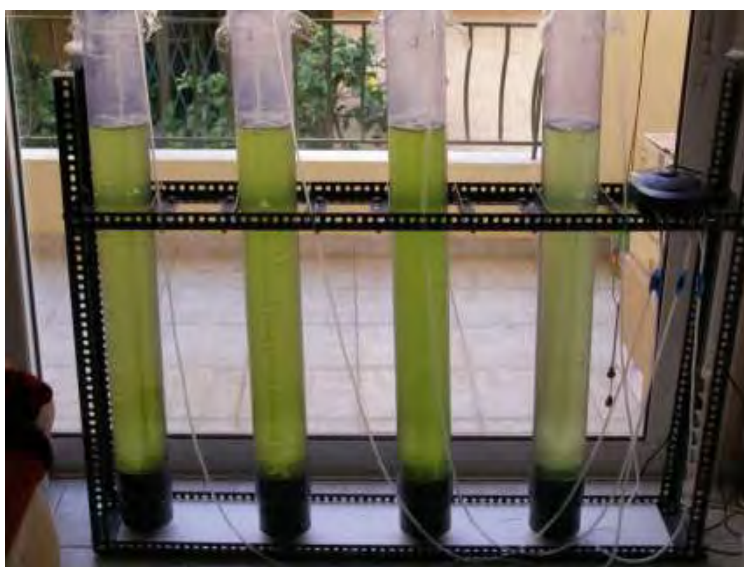
Εικόνα 36. Τέσσερις PBRs με 7 L καλλιέργειας ο κάθε ένας.
