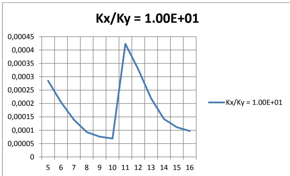
Εικόνα 33: Γραφική απεικόνιση συνδυαστικών αποτελεσμάτων για K_x/K_y=1.00E+01 .
