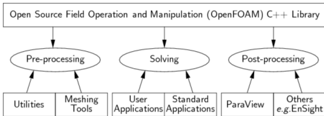
Εικόνα 8: Επισκόπηση λειτουργίας του OpenFOAM. 7
