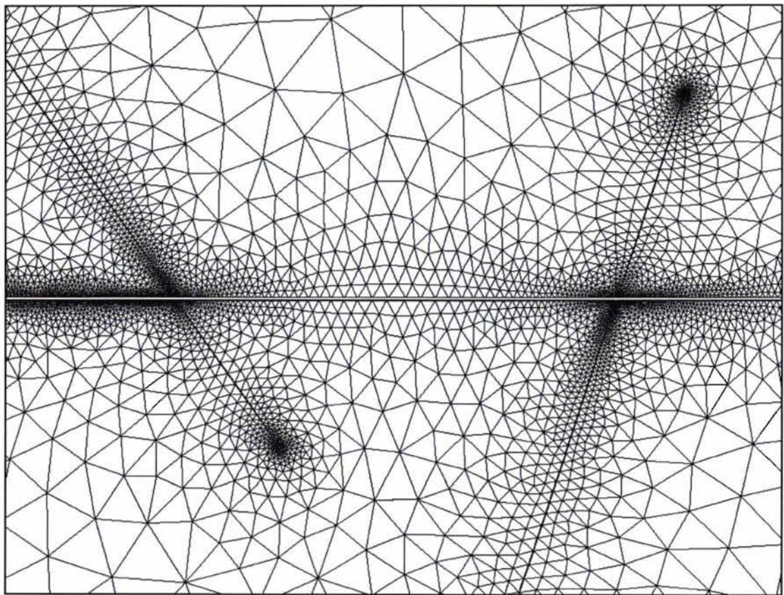
Σχ. 63 – Τυπική λεπτομέρεια πλέγματος περιοδικής γεωμετρίας, \alpha=1000 , \alpha_f=1 , \theta=0 , \epsilon=\pi/2
