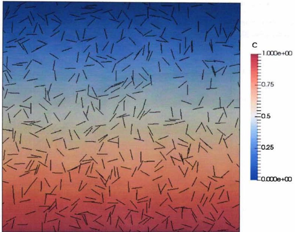
Σχ. 64 – Τυπικό διάγραμμα συγκεντρώσεων για \alpha=1000 , \alpha\phi=1 , \theta=0 , \epsilon=\pi/2
