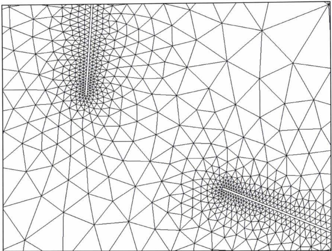
Σχ. 62 – Τυπική λεπτομέρεια πλέγματος, \alpha=1000 , \alpha_f=1 , \theta=0 , \epsilon=\pi/2
