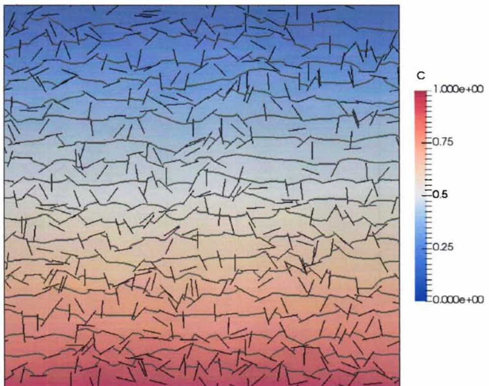
Σχ. 65 – Τυπικό διάγραμμα ισουψών συγκέντρωσης (20 ισουψείς ανά 0.05), για \alpha=1000 , \alpha\phi=1 , \theta=0 , \epsilon=\pi/2
