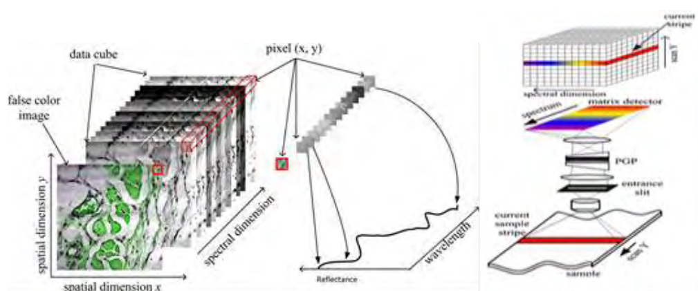
Εικόνα 4. Υπερφασματικός κύβος ενός υπερφασματικού αισθητήρα απεικόνισης (αριστερά), Pushbroom σύστημα σάρωσης (δεξιά). Φωτογραφίες που ελήφθησαν από τους Li et al., (2013) .
