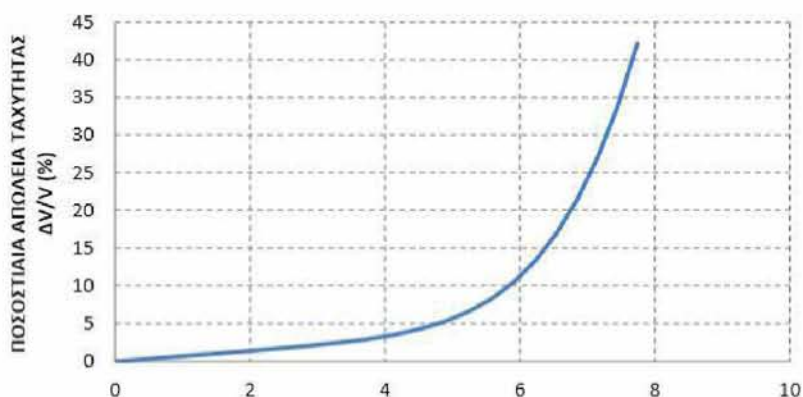
Διάγραμμα μείωσης ταχύτητας – Ένταση ανέμου.
