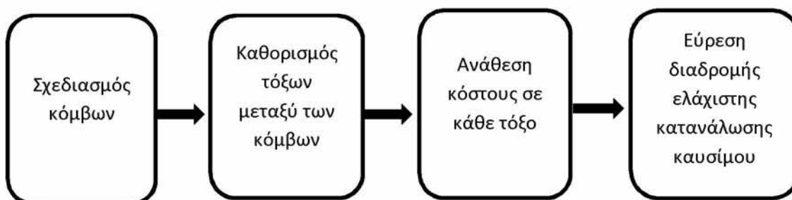
Σχήμα 6.4 Αλγόριθμος δρομολόγησης
