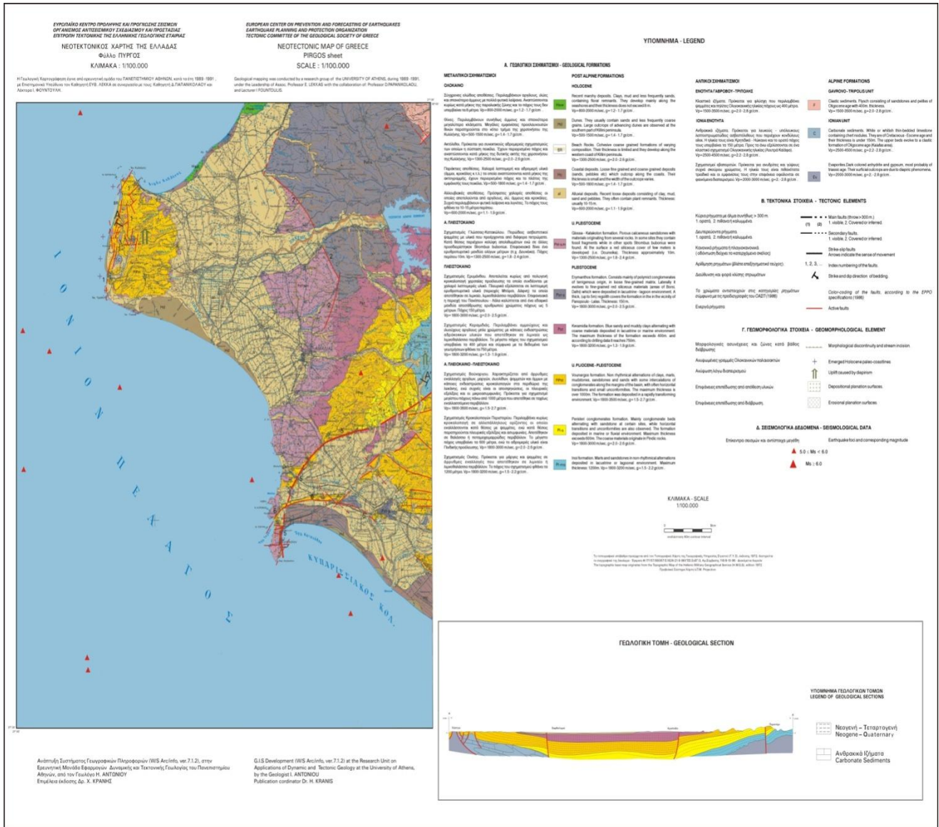
Σχήμα 12 : Γεωλογικός χάρτης «Φύλλο Πύργου» Πηγή : Lekkas, E., Paranikolaou, D., Fountoulis, I., 1992.
