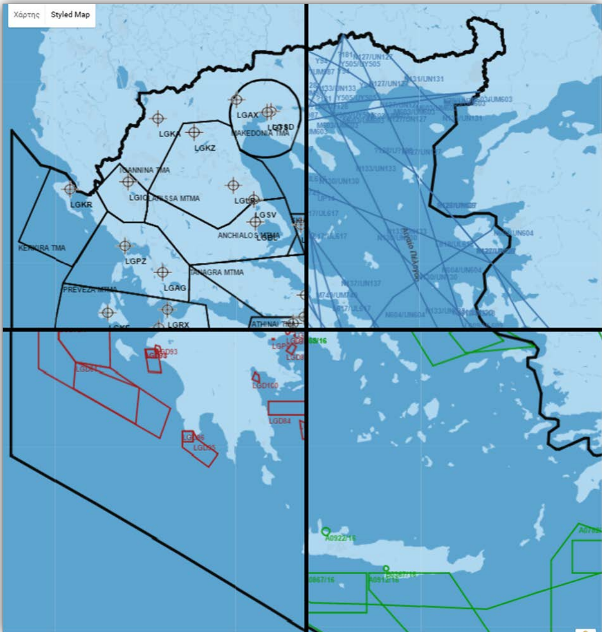
Εικόνα 35. Πάνω αριστερά απεικονίζονται αεροδρόμια και τερματικές περιοχές ελέγχου, πάνω δεξιά αεροδιάδρομοι, κάτω αριστερά πεδία βολής και κάτω δεξιά αγελιές.
