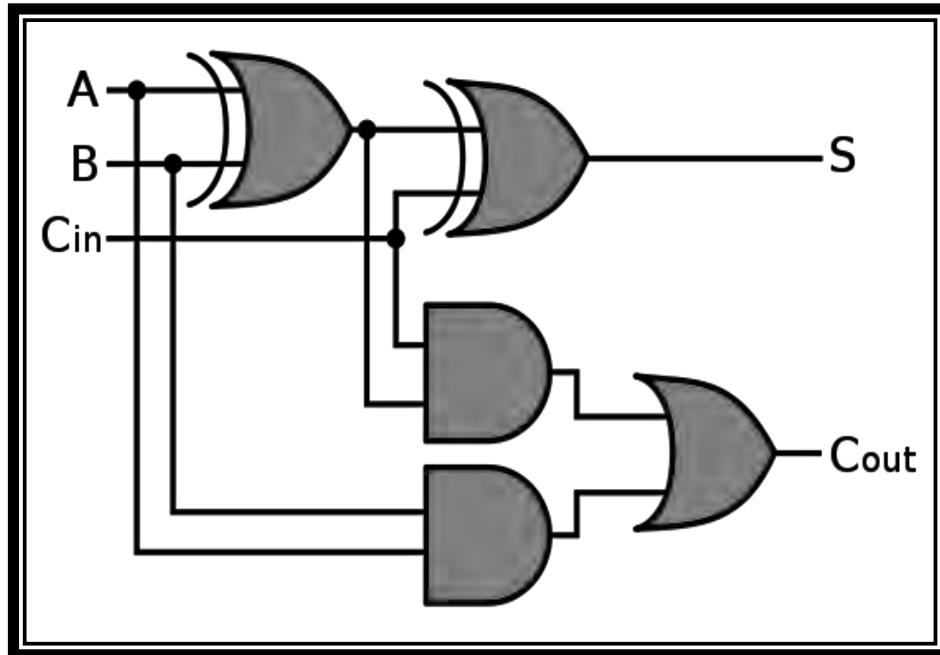
Εικόνα 10 Fulladder
