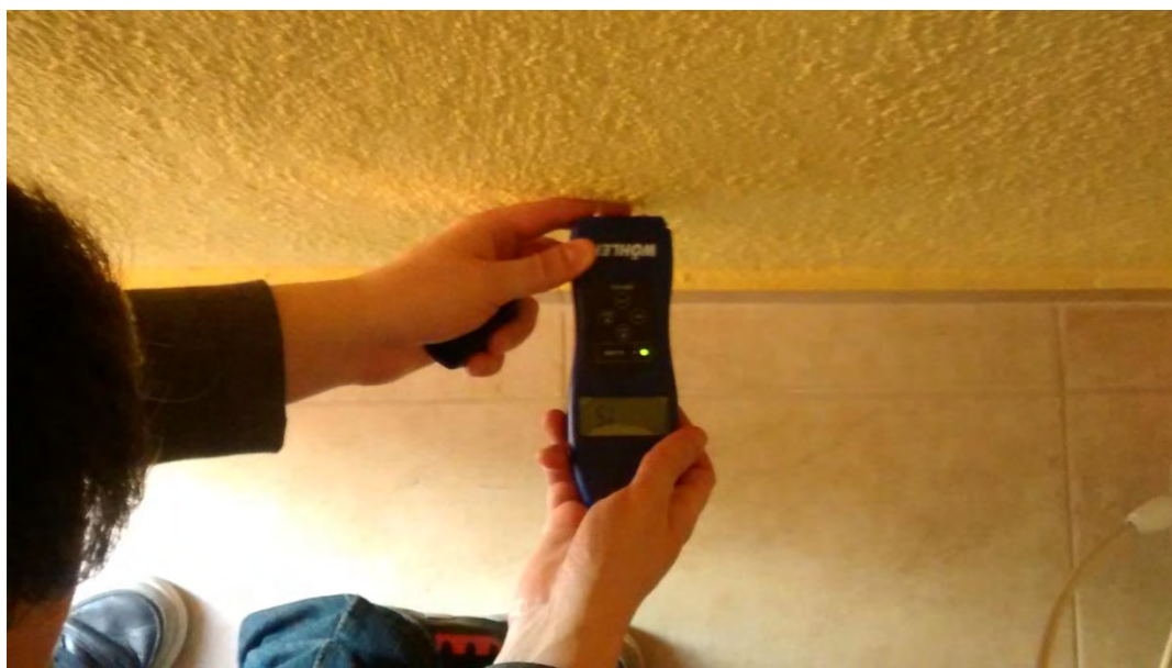
Εικόνα 67: Φωτογραφία που λήφθηκε κατά τη διάρκεια μιας μέτρησης υγρασίας όπου διακρίνονται οι βελόνες που εισχωρούν στο τείχο.
