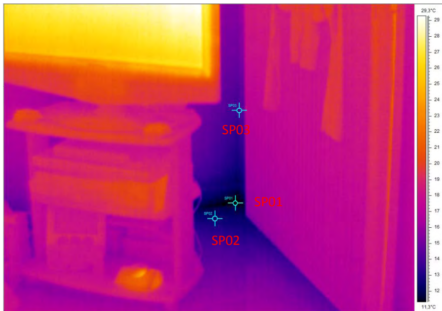
Εικόνα 105: Υπέρυθρη φωτογραφία της νοτιοανατολικής γωνίας στο καθιστικό της οικίας όπου είναι εμφανής μια έντονη θερμοκρασιακή διαφορά στην περιοχή πιθανώς λόγω ελλιπούς μόνωσης.
