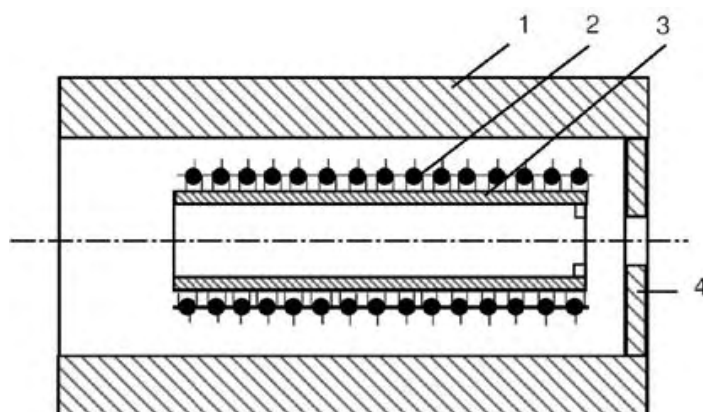
Εικόνα 14: Σχηματική απεικόνιση ενός πραγματικού «μέλαν σώματος» όπου 1-κερμαϊκός αγωγός, 2-θερμαντικά στοιχεία, 3-αγωγός από Al_2O_3 , 4-άνοιγμα
