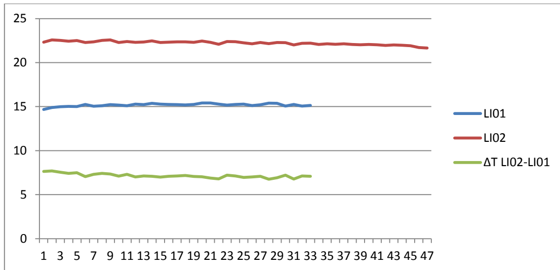
Διάγραμμα 12: Τα θερμοκρασιακά προφίλ κατά μήκος των γραμμών που έχουν επισημανθεί στην εικόνα 103 και η μεταβολή της θερμοκρασιακής διαφοράς των LI02-LI01.
