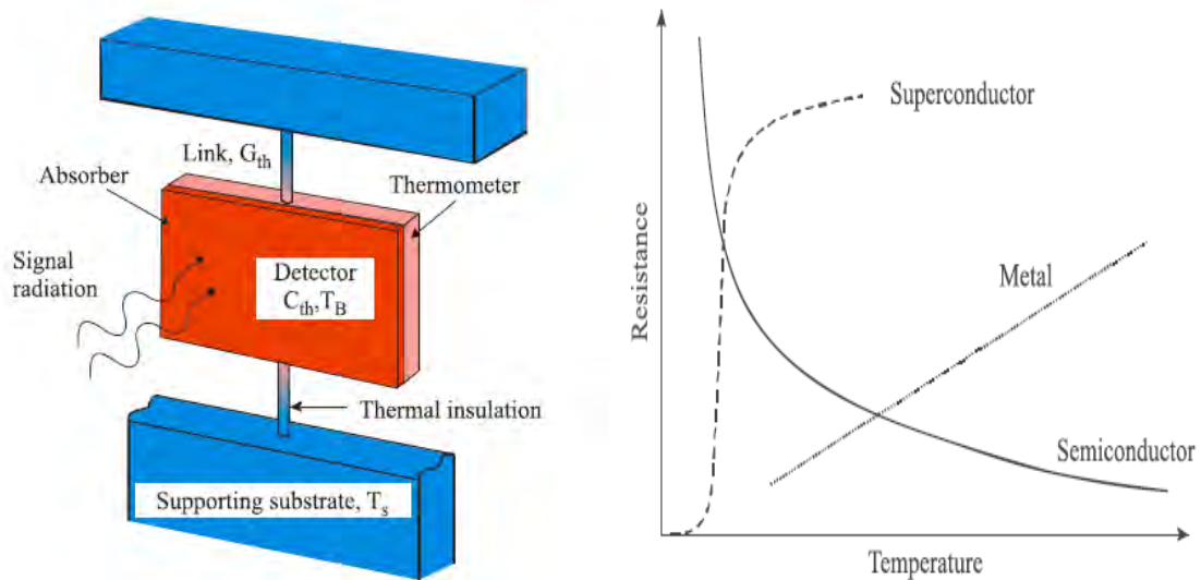
Εικόνα 29: Σχηματική αναπαράσταση ενός θερμικού αισθητήρα (αριστερά) – Μεταβολή της αντίστασης συναρτήσει της θερμοκρασίας για τρία υλικά κατασκευής βολομέτρων.
