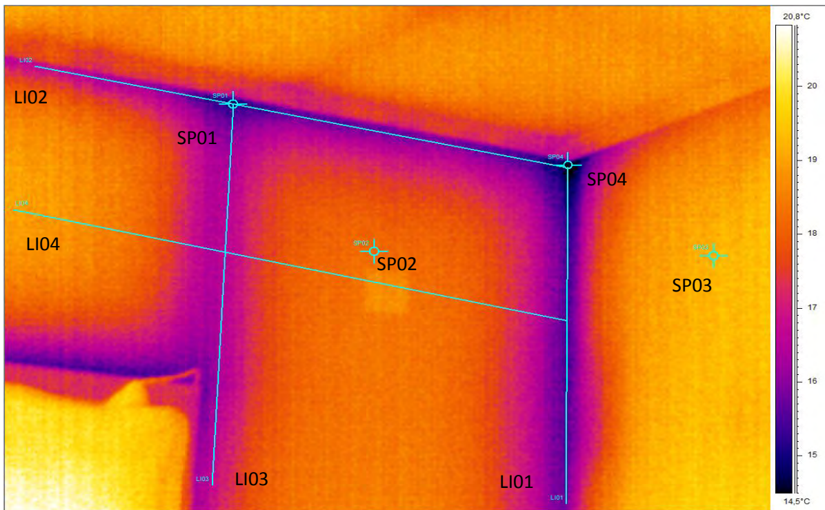
Εικόνα 93: Υπέρυθρη λήψη από τον δυτικό τοίχο του κλιμακοστασίου. Διακρίνεται ευκρινώς ο μεταλλικός σκελετός του κτιρίου.
