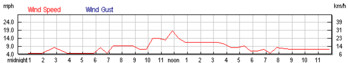
Εικόνα 52: Μεταβολή της ταχύτητας του ανέμου κατά τη διάρκεια της ίδιας ημέρας.
