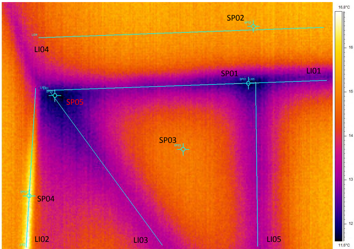
Εικόνα 102: Υπέυρυθρη φωτογραφία του παραπάνω τοίχου.
