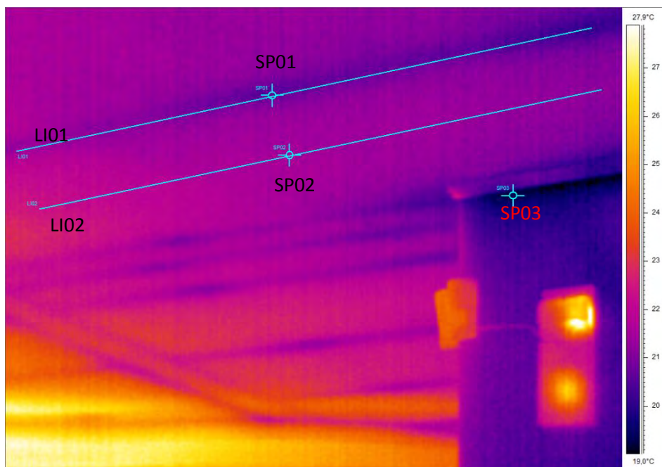
Εικόνα 104: Υπέρουθρη φωτογραφία της οροφής της κουζίνας. Είναι εμφανείς οι μεταλλικές δοκοί του σκελετού της οροφής.
