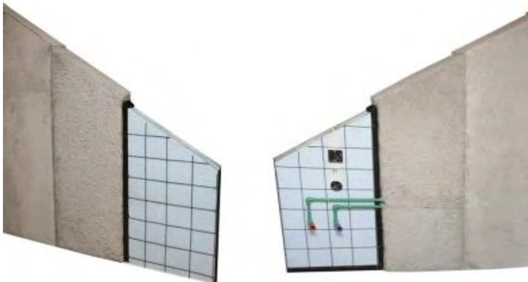
Εικόνα 43: Φωτογραφία των διάφορων σταδίων κατασκευής της τοιχοποιίας όπου φαίνονται τα στρώματα επιχρίσματος.
