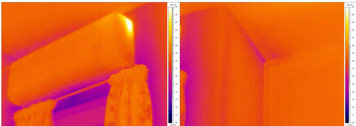
Εικόνα 80: Υπέρυθρες φωτογραφίες από τον δυτικό και νότιο τοίχο του δωματίου Η/Υ.
