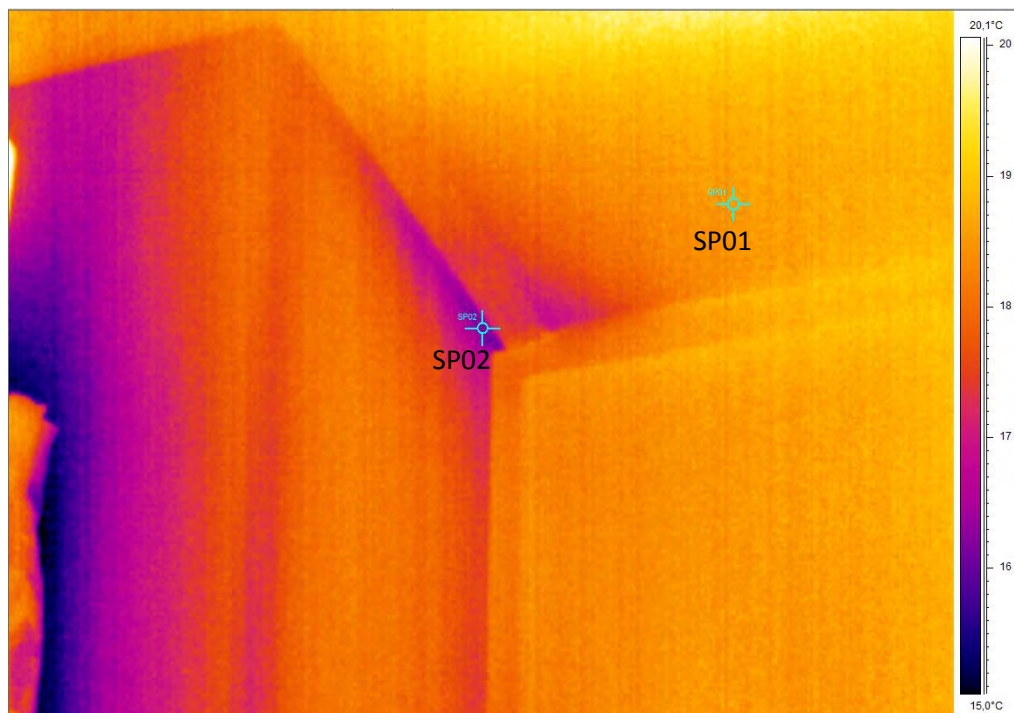
Εικόνα 106: Υπέυρθη φωτογραφία του νότιου τοίχου στο δωμάτιο του Η/Υ όπου φαίνεται ένα πιθανό σημείο ελλιπούς μόνωσης.
