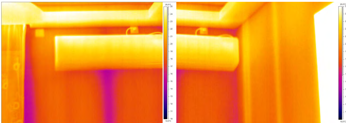
Εικόνα 81: Υπέρυθρες φωτογραφίες από τον ανατολικό και νότιο τοίχο του καθιστικού.
