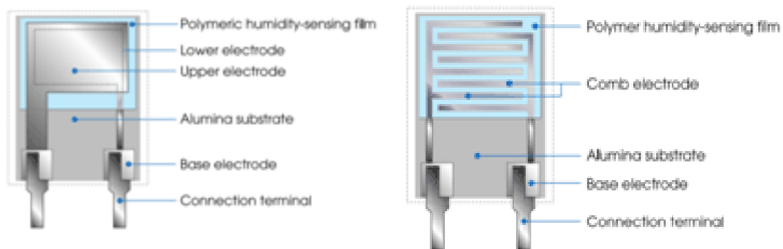
Εικόνα 66: Σχηματική απεικόνιση των δυο αισθητήρων υγρασίας που διαθέτει το υγρασιόμετρο ένας για κάθε τρόπο μέτρησης της υγρασίας.
