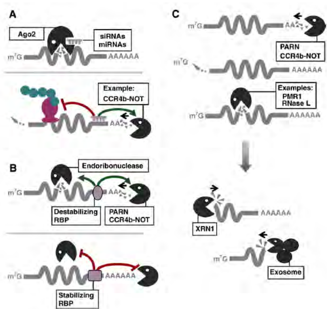
Εικόνα 14. Τρόποι δράσης trans-δραστικών παραγόντων όπως Α. μη κωδικά RNAs, Β. RNA-συνδεόμενες πρωτεΐνες (RBP) και C. ριβονουκλεάσες στη ρύθμιση της σταθερότητας των mRNAs (Kim and Lee, 2009)
