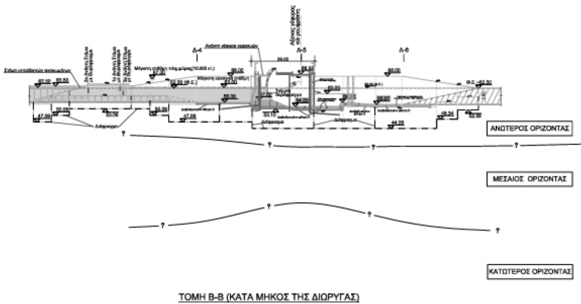
Σχέδιο 3: Τομές ρουφράκτη
