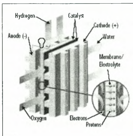
Εικόνα 18: Κύρια μέρη μιας κυψέλης καυσίμου (Κάππος, 2009)
