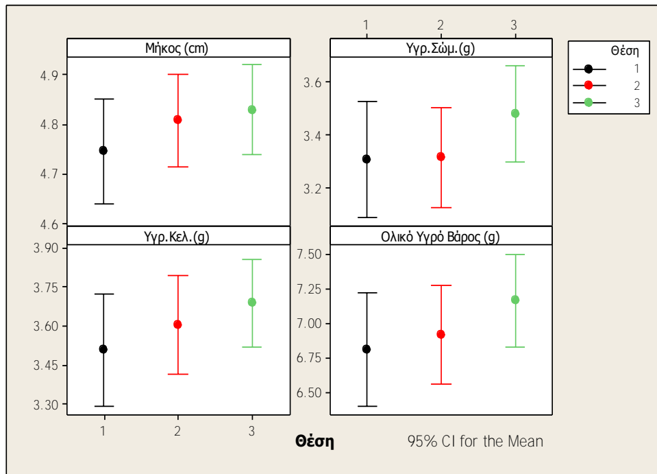
Εικ.3.8 Κατά βάθος μεταβολή των μέσων τιμών του μήκους, και του υγρού βάρους σώματος, κελύφους και ολικού των μυδιών στο σταθμό μελέτης.
