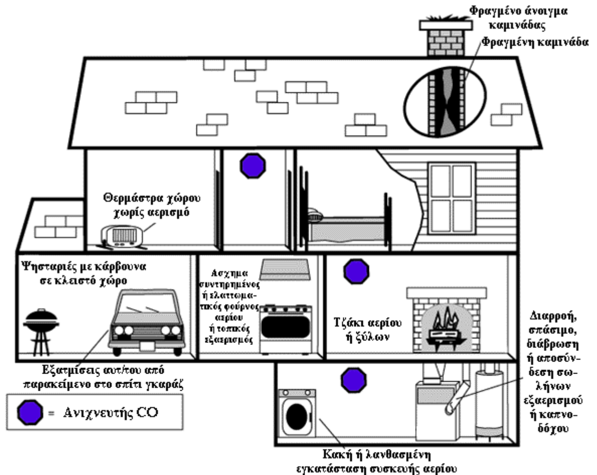
Σχήμα 3.1 : Ατελής καύση
