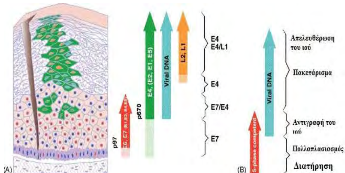
Εικόνα 19: Μεταγραφή του ιικού γενώματος.
