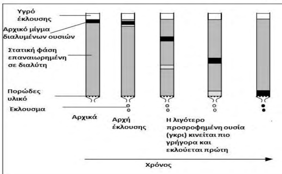
Σχήμα 14. Χρωματογραφία στήλης.
