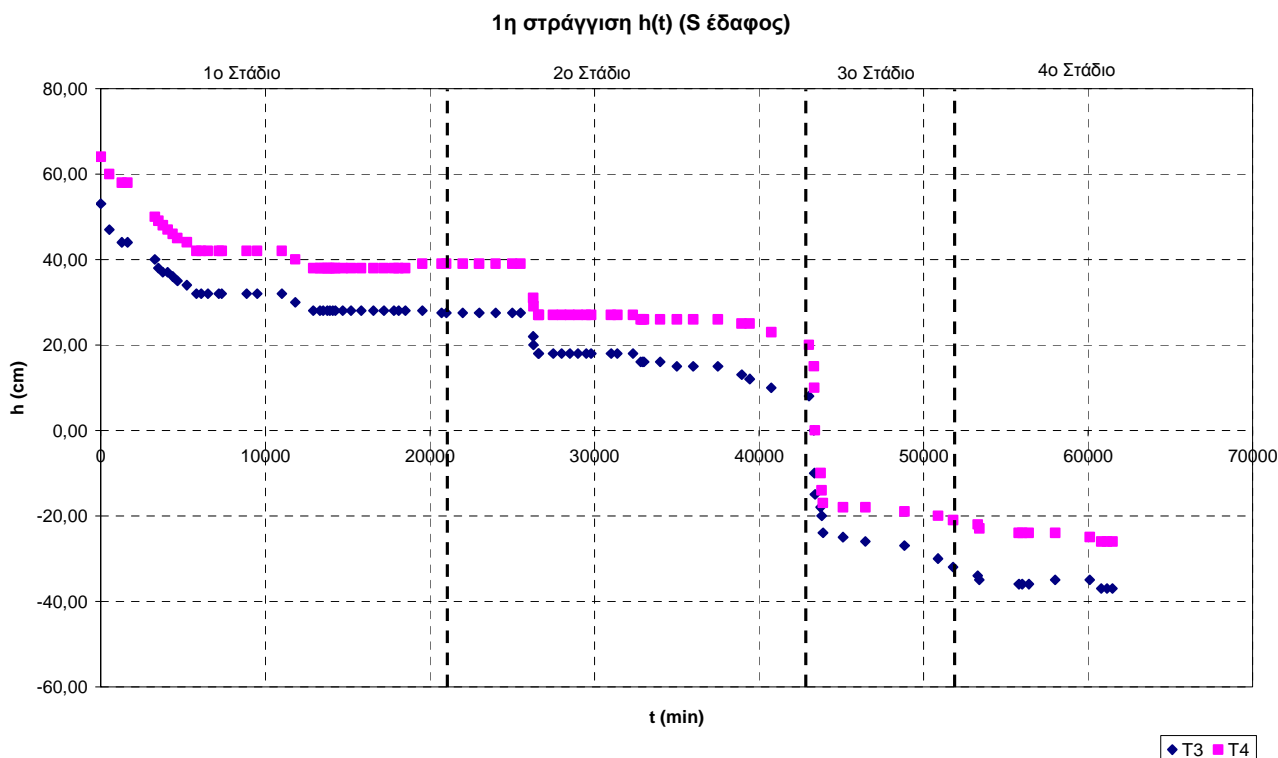
Σχήμα 3.18 Πειραματικές τιμές της πίεσης ως προς το χρόνο στο αμμώδες έδαφος (κάτω στρώση), κατά την 1 η στράγγιση
