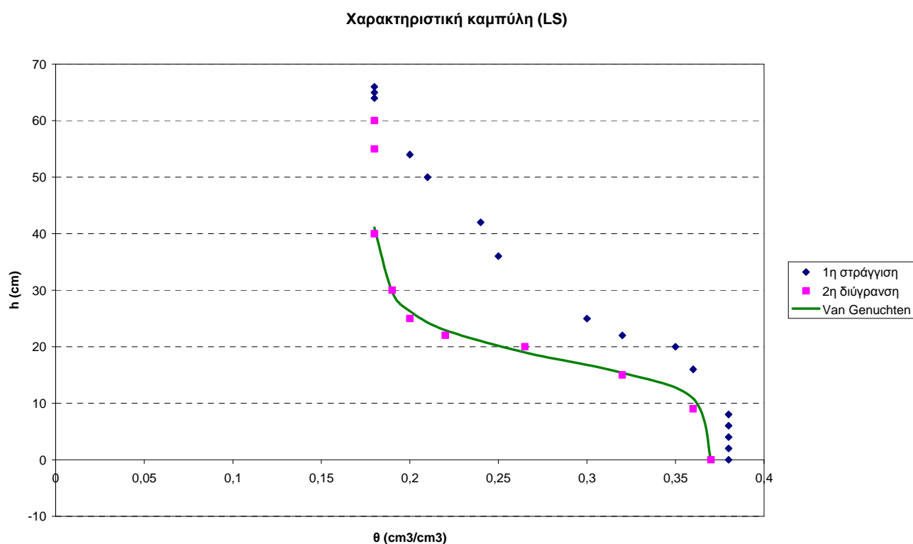
Σχήμα 4.1 Χαρακτηριστικές καμπύλες για το ηλοαμμώδες (LS) έδαφος-προσομοίωση 2ης διύγρανσης με μοντέλο van Genuchten
