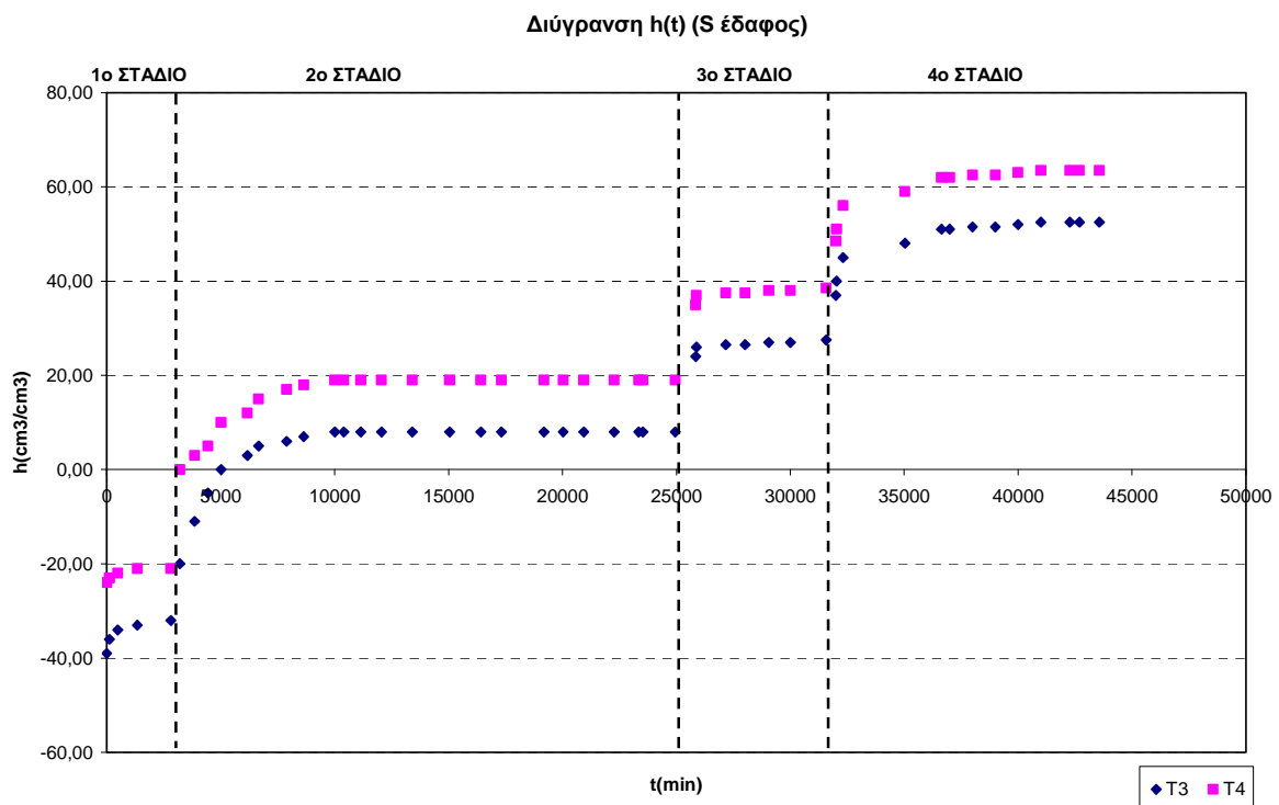
Σχήμα 3.22 Πειραματικές τιμές της πίεσης ως προς το χρόνο στο αμμώδες έδαφος (κάτω στρώση), κατά τη 2 η διύγνωση
