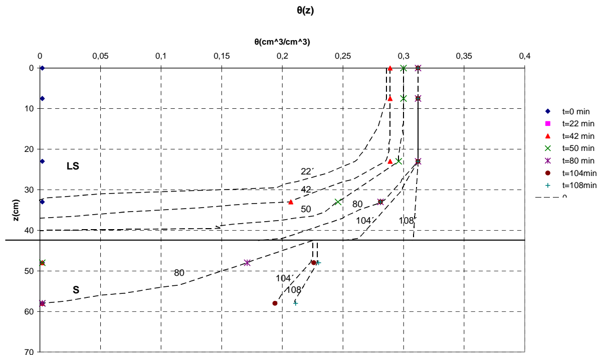
Σχήμα 3.10 Εδαφική υγρασία σε συνάρτηση με το βάθος, (μέτωπα εδαφικής υγρασίας)
