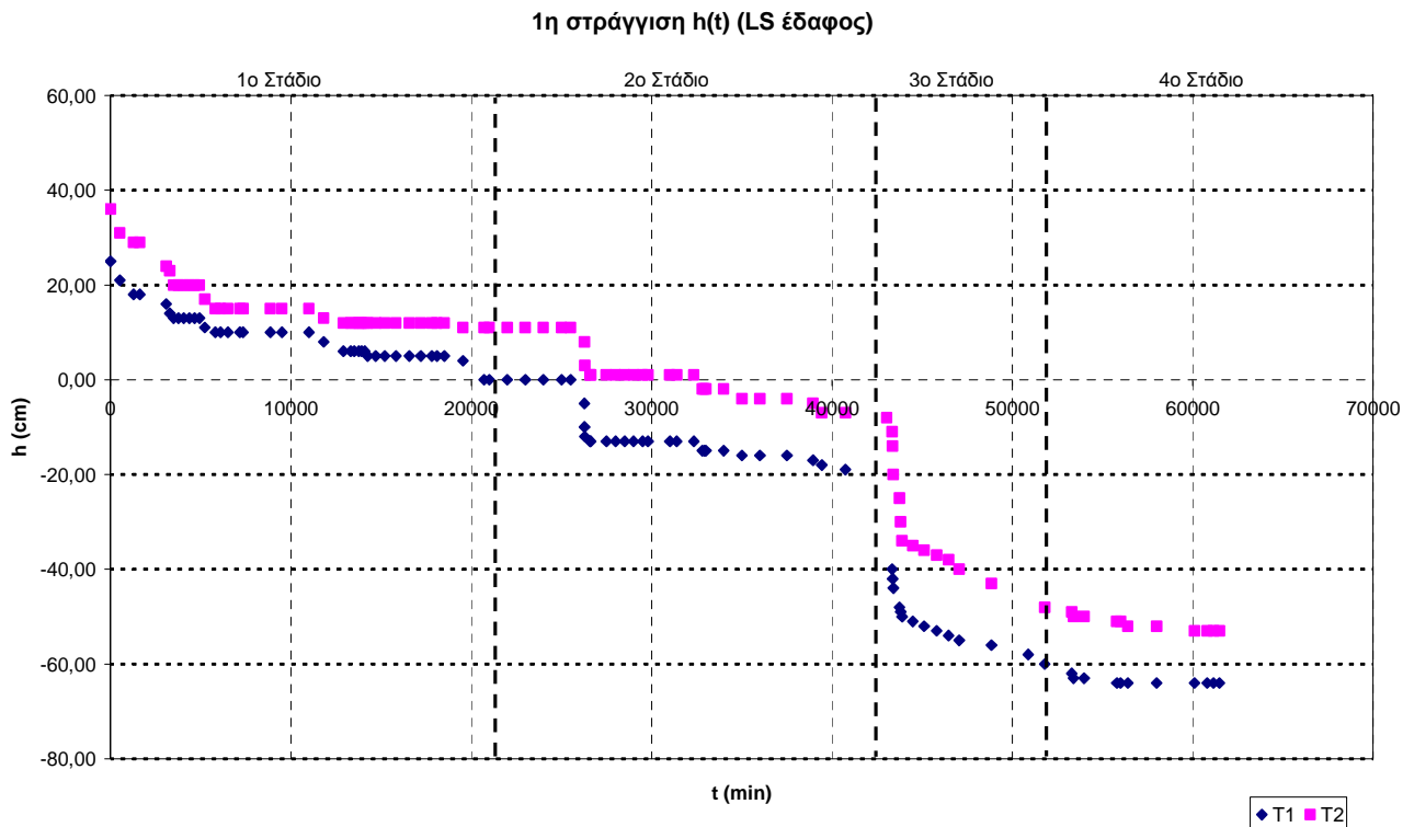
Σχήμα 3.17 Πειραματικές τιμές της πίεσης ως προς το χρόνο στο πηλοαμμώδες έδαφος (πάνω στρώση), κατά την 1 η στράγγιση
