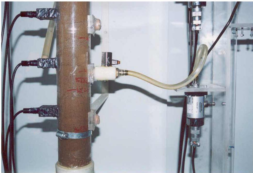
Εικόνα 2.5 Σύστημα κεραμικής κάψας – δεξαμενής νερού – εύκαμπτου σωλήνα όταν ήδη έχει συνδεθεί με την εδαφική στήλη και το μετατροπέα πίεσης (Αγγελάκη, 2004).
