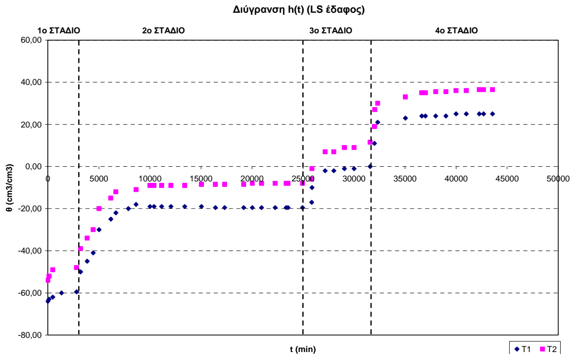
Σχήμα 3.21 Πειραματικές τιμές της πίεσης ως προς το χρόνο στο πηλοαμμώδες έδαφος (πάνω στρώση), κατά τη 2 η διύγρανση
