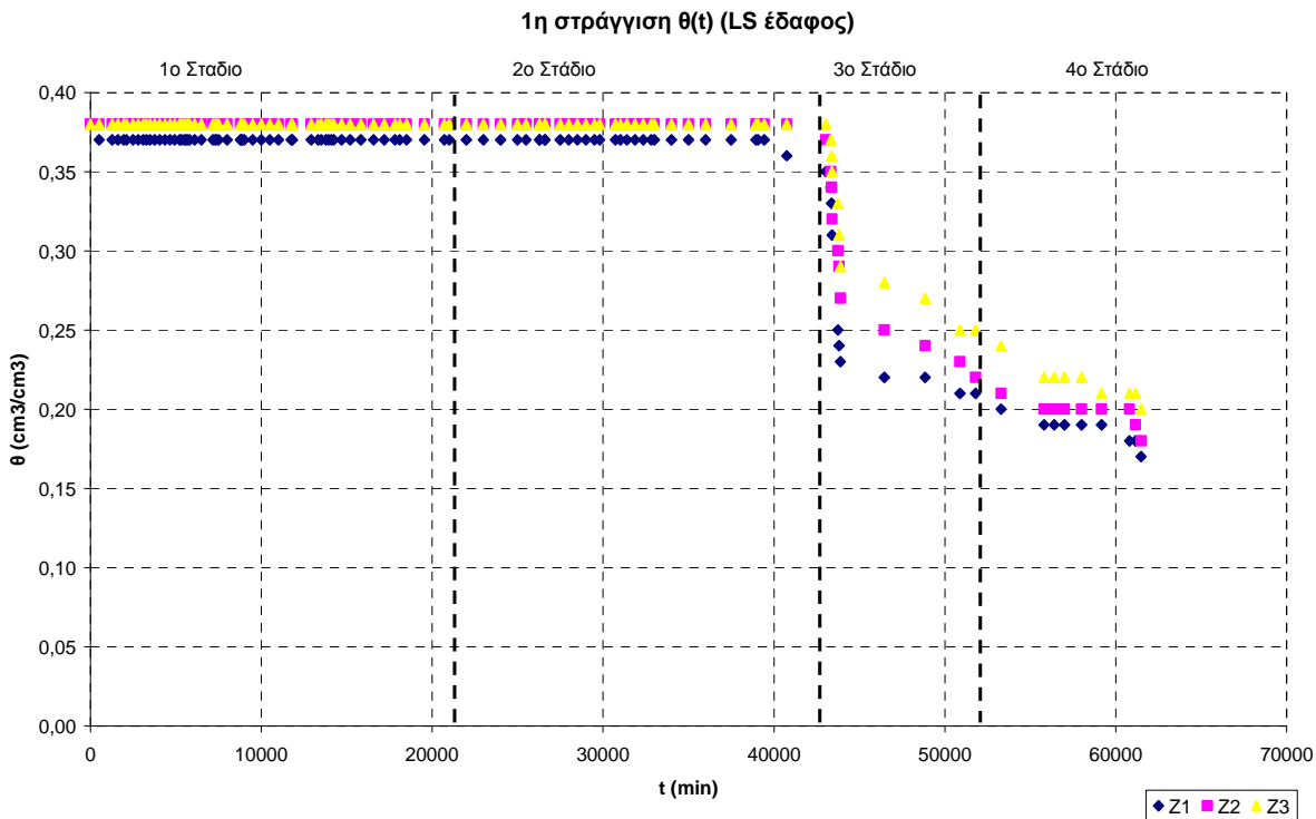
Σχήμα 3.15 Πειραματικές τιμές της υγρασίας ως προς το χρόνο στο πηλοαμμώδες έδαφος (πάνω στρώση), κατά την 1 η στράγγιση.
