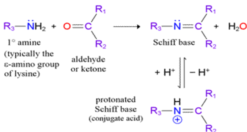
Εικόνα 17: Παράδειγμα πυρηνόφιλης προσθήκης προς σχηματισμό βάσης Schiff.
