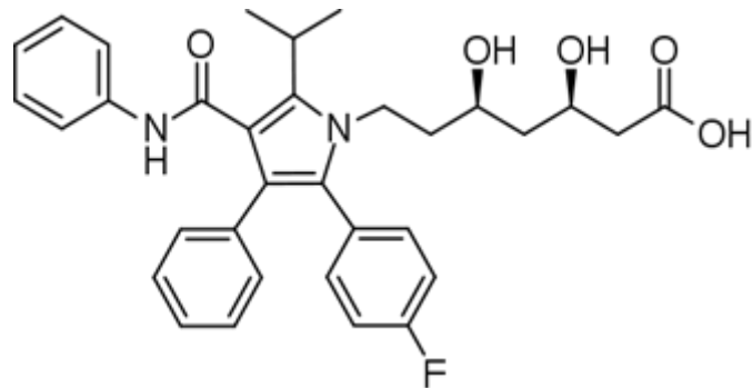
Εικόνα 8: Μοριακή δομή του Atorvastatin
