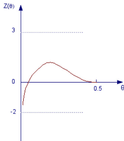
Γράφημα 3: -2 < z(\theta) < 3
