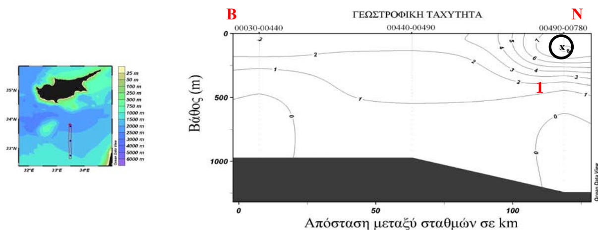
Εικόνα 3.5.4.11: Εγκάρσια τομή AA9 των γεωστροφικών ρευμάτων της ευρύτερης περιοχής της Λεβαντινής λεκάνης
