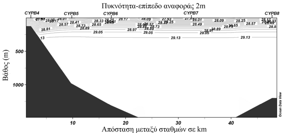
Εικόνα 3.1.2.56: Εγκάρσια τομή της πυκνότητα – A10
