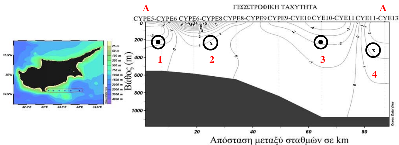
Εικόνα 3.5.3.5: Εγκάρσια τομή A3 των γεωστροφικών ρευμάτων στην νοτιοανατολική Λεβαντινή.
