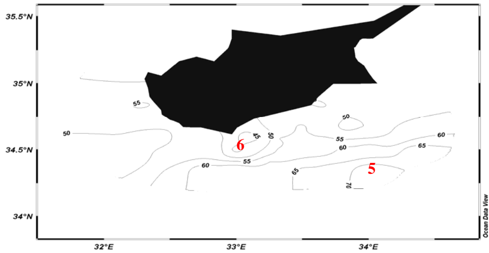
Εικόνα 3.3.13: Τοπογραφία της ισόπυκνης επιφάνειας των 28,4 \text{ kg/m}^3
