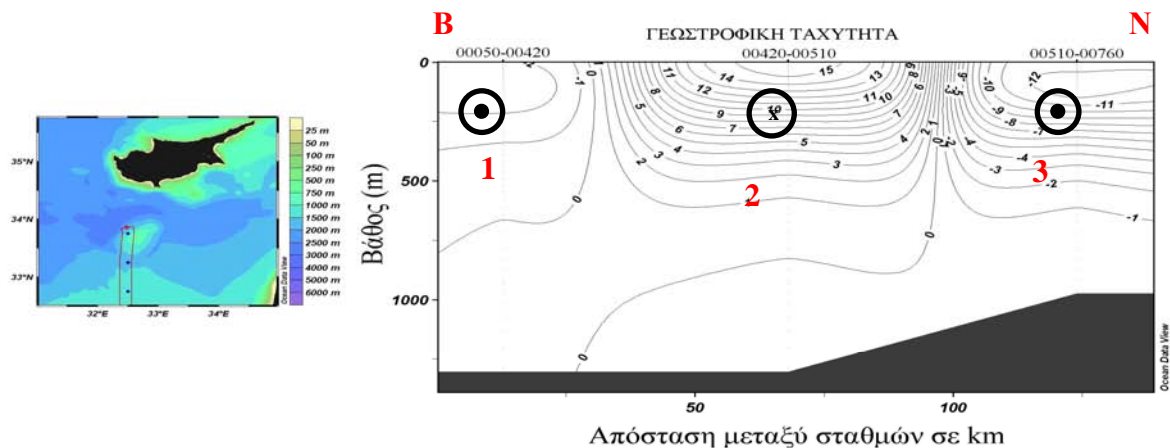
Εικόνα 3.5.4.10: Εγκάρσια τομή AA8 των γεωστροφικών ρευμάτων της ευρύτερης περιοχής της Λεβαντινής λεκάνης.
