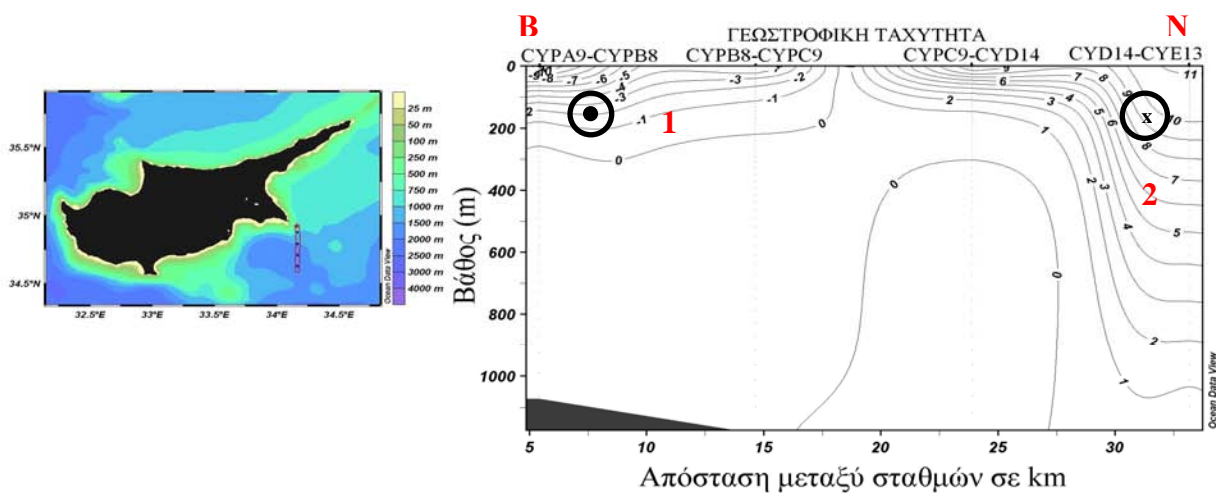
Εικόνα 3.5.3.14: Εγκάρσια τομή ΑΑ5 των γεωστρωφικών ρευμάτων στην νοτιοανατολική Λεβαντινή.
