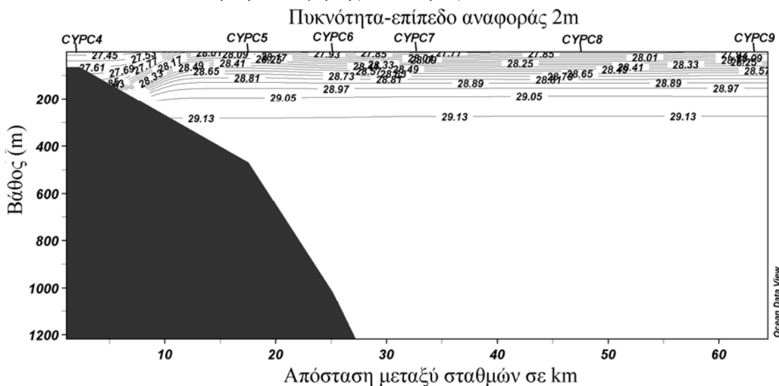
Εικόνα 3.1.2.62: Εγκάρσια τομή της πυκνότητας – Α11
