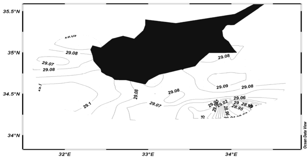
Εικόνα 3.1.1.12: Επιφανειακή κατανομή της δυναμικής πυκνότητας Rev.Level (2 m) – (200 m)
