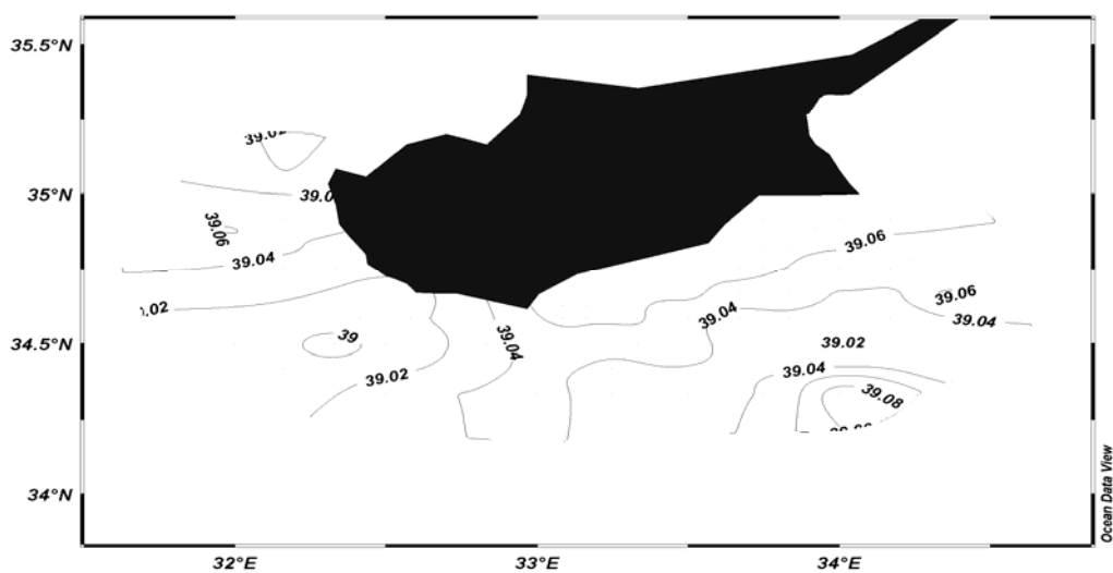
Εικόνα 3.1.1.11: Οριζόντια κατανομή της αλατότητας (200 m)
