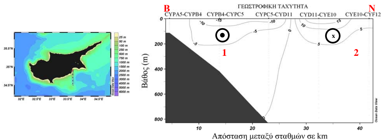
Εικόνα 3.5.3.12: Εγκάρσια τομή ΑΑ3 των γεωστρωφικών ρευμάτων στην νοτιοανατολική Λεβαντινή.
