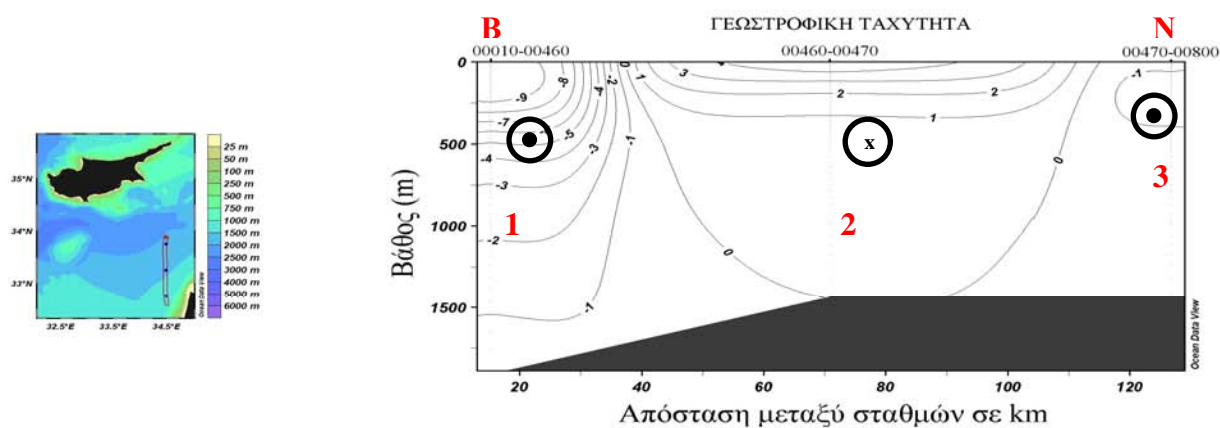
Εικόνα 3.5.4.12: Εγκάρσια τομή AA10 των γεωστροφικών ρευμάτων της ευρύτερης περιοχής της Λεβαντινής λεκάνης.
