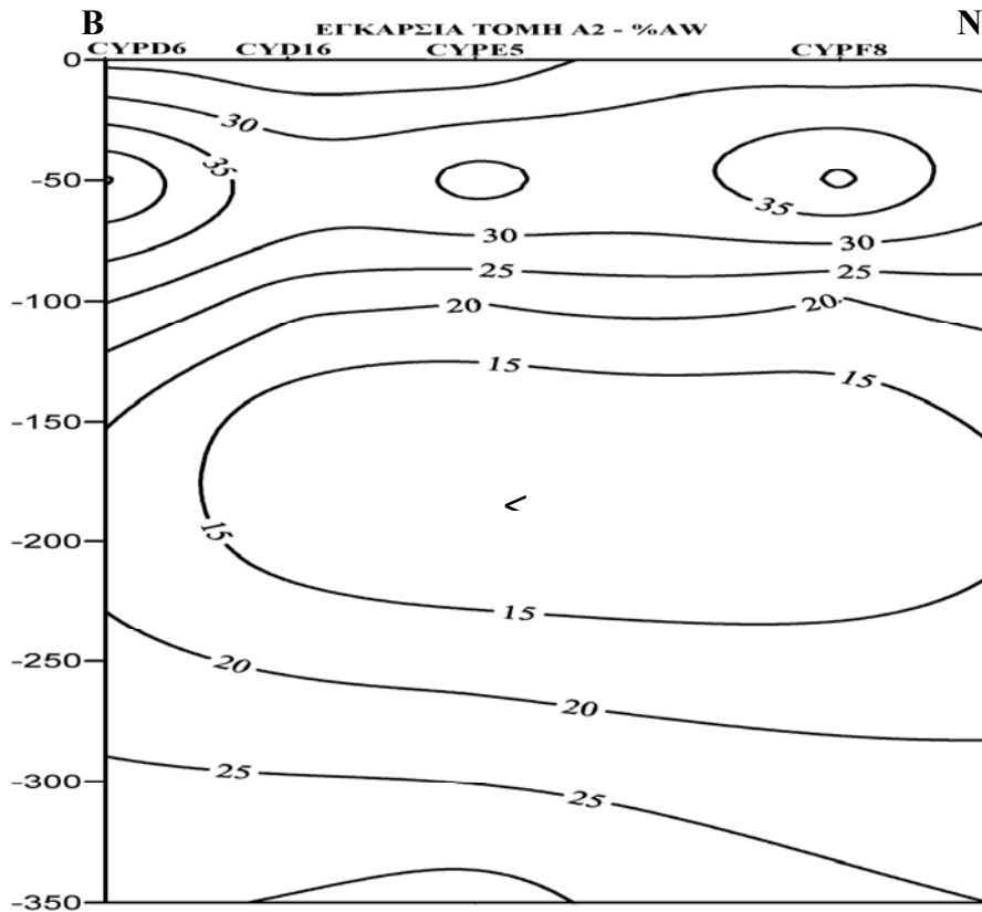
Εικόνα 3.4.2.4: Ποσοστό συμμετοχής του MAW κατά μήκος της τομής Α2.
