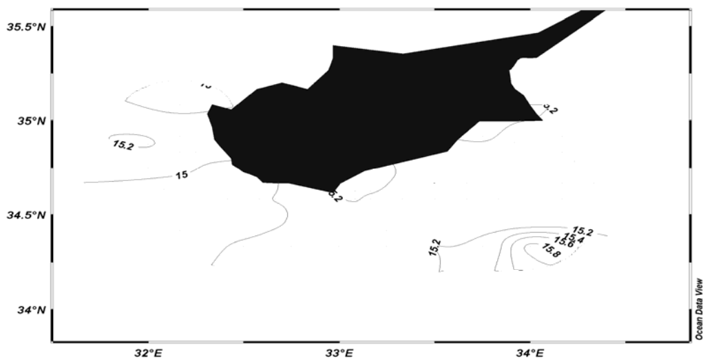
Εικόνα 3.1.1.10: Οριζόντια κατανομή της δυναμικής θερμοκρασίας Rev.Level (2 m) – (200 m)
