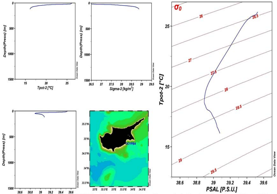
PSAL [P.S.U.] Σταθμός CYPB4, Τέλος Καλοκαιριού του 1995 (Δυναμική θερμοκρασία, αλατότητα, δυναμική πυκνότητα και διάγραμμα T-S).
