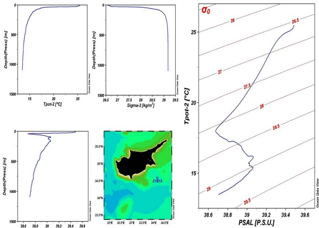
PSAL [P.S.U.] Σταθμός CYE13, Τέλος Καλοκαιριού του 1995 (Δυναμική θερμοκρασία, αλατότητα, δυναμική πυκνότητα και διάγραμμα T-S).
