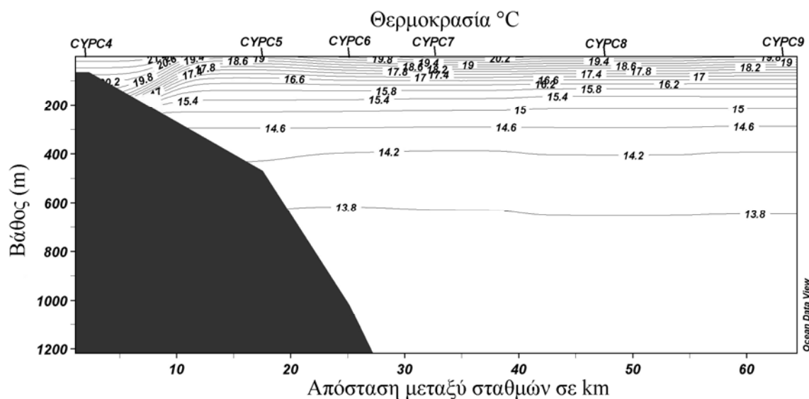
Εικόνα 3.1.2.60: Εγκάρσια τομή θερμοκρασίας-Α11
