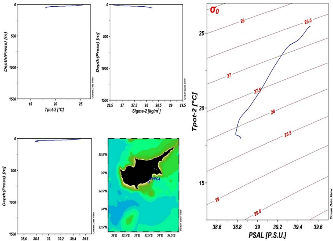
PSAL [P.S.U.] Σταθμός CYPC4, Τέλος Καλοκαιριού του 1995 (Δυναμική θερμοκρασία, αλατότητα, δυναμική πυκνότητα και διάγραμμα T-S).
