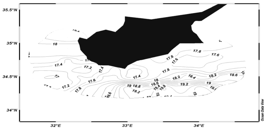
Εικόνα 3.1.1.4: Οριζόντια κατανομή της δυναμικής θερμοκρασίας Rev.Level (2 m) – (50 m)
