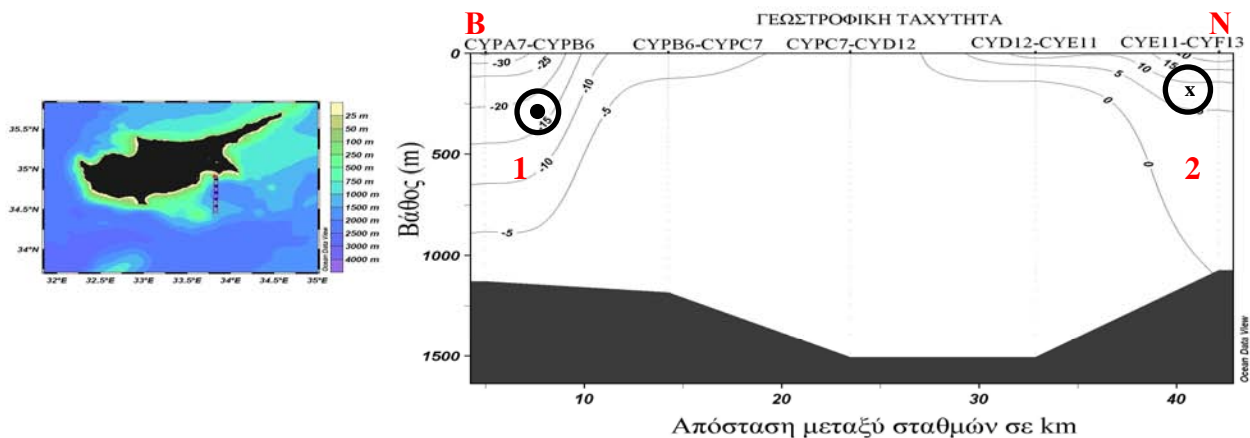
Εικόνα 3.5.3.13: Εγκάρσια τομή ΑΑ4 των γεωστρωφικών ρευμάτων στην νοτιοανατολική Λεβαντινή.
