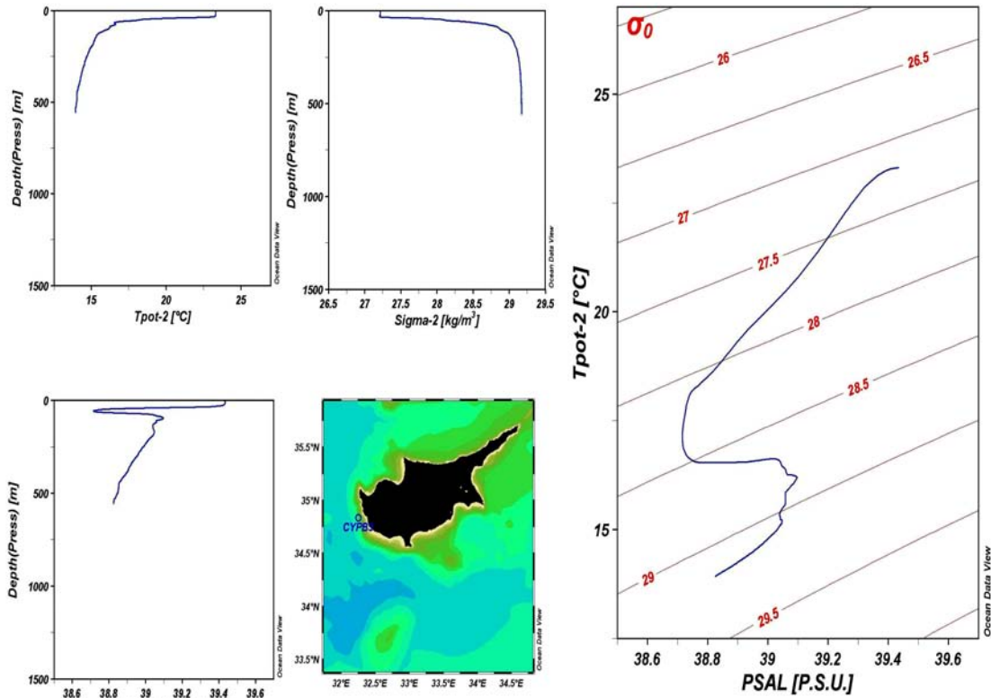
PSAL [P.S.U.] Σταθμός CYB3, Τέλος Καλοκαιριού του 1995 (Δυναμική θερμοκρασία, αλατότητα, δυναμική πυκνότητα και διάγραμμα T-S).
