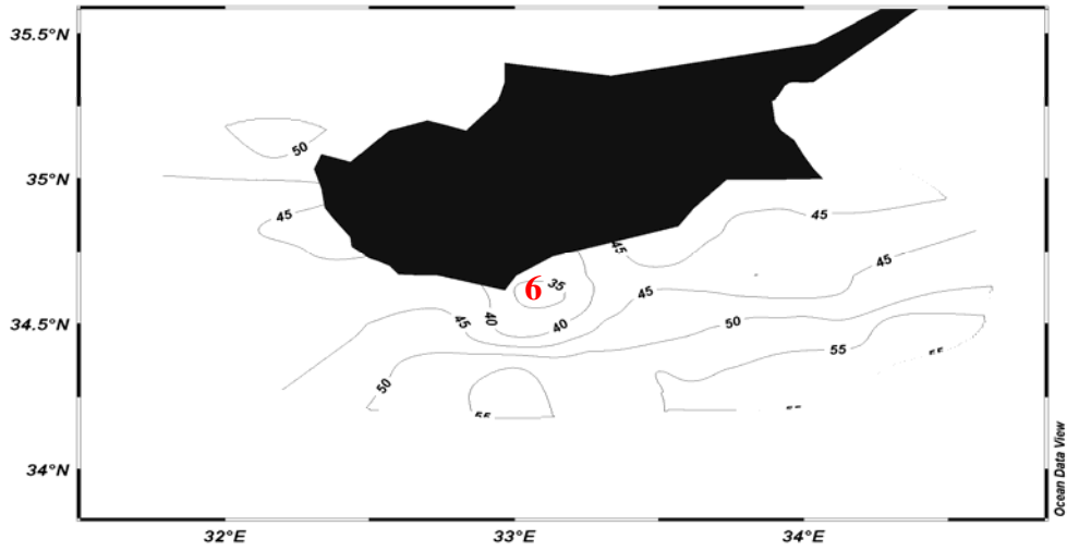
Εικόνα 3.3.16: Τοπογραφία της ισόπυκνης επιφάνειας των 28,2 \text{ kg/m}^3
