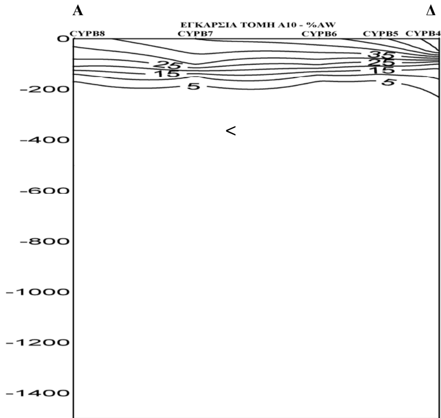
Εικόνα 3.4.2.20: Ποσοστό συμμετοχής του ΜΑW κατά μήκος της τομής Α10
