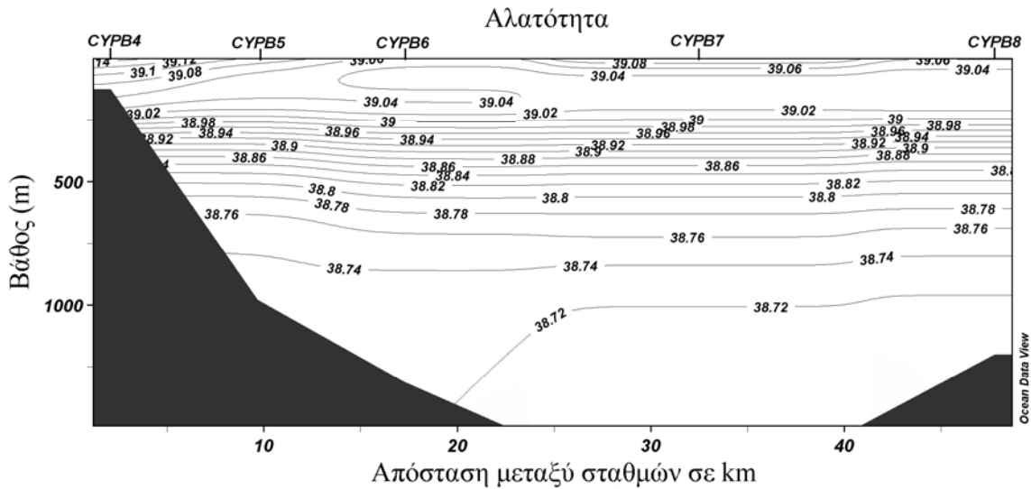
Εικόνα 3.1.2.55: Εγκάρσια τομή της αλατότητας – A10
