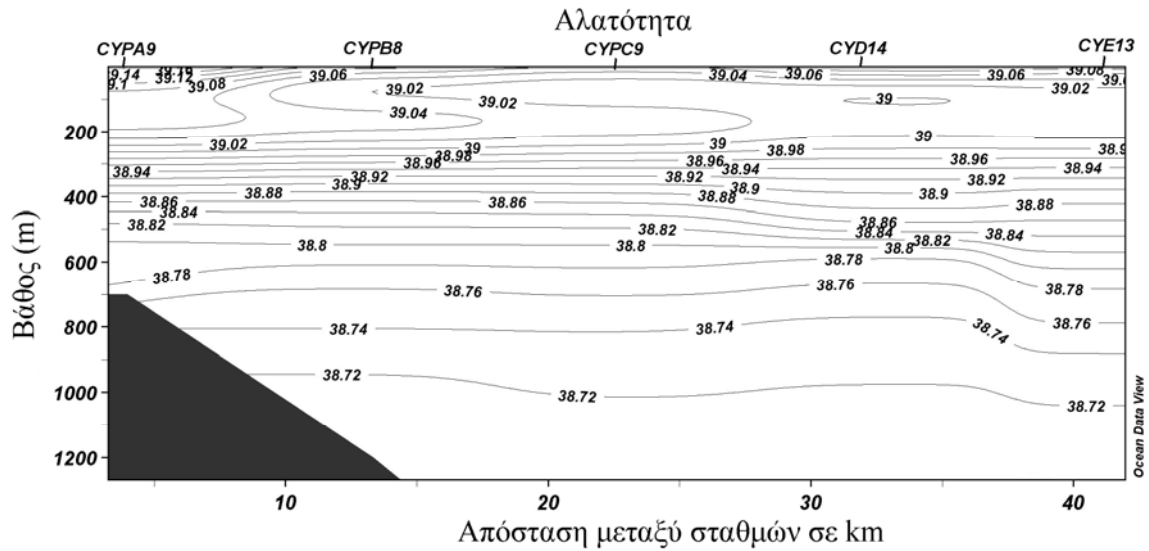
Εικόνα 3.1.2.43: Εγκάρσια τομή της αλατότητας – Α8
