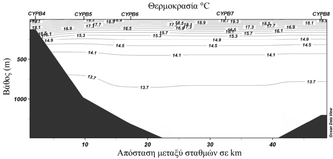
Εικόνα 3.1.2.54: Εγκάρσια τομή θερμοκρασίας-A10
