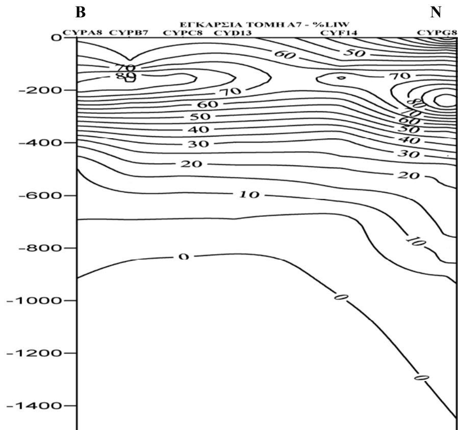
Εικόνα 3.4.2.15: Ποσοστό συμμετοχής του LIW κατά μήκος της τομής A7
