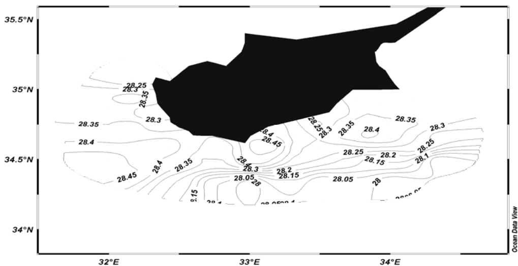
Εικόνα 3.1.1.6: Επιφανειακή κατανομή της δυναμικής πυκνότητας Rev.Level (2 m) – (50 m)
