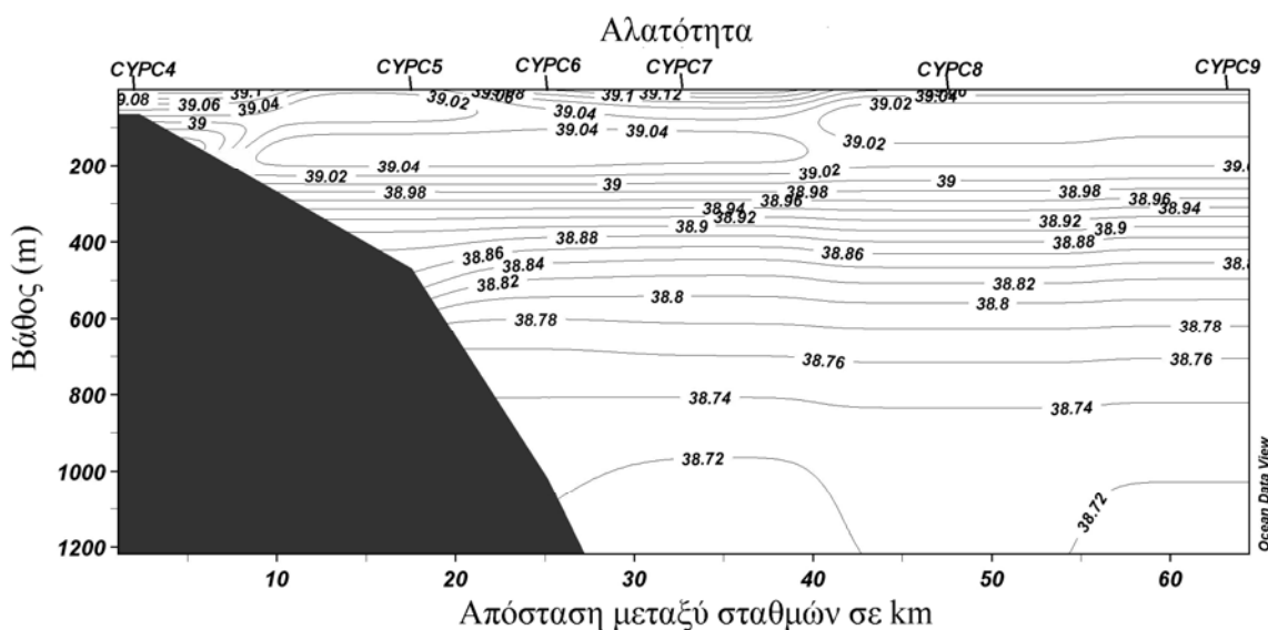
Εικόνα 3.1.2.61: Εγκάρσια τομή της αλατότητας – Α11
