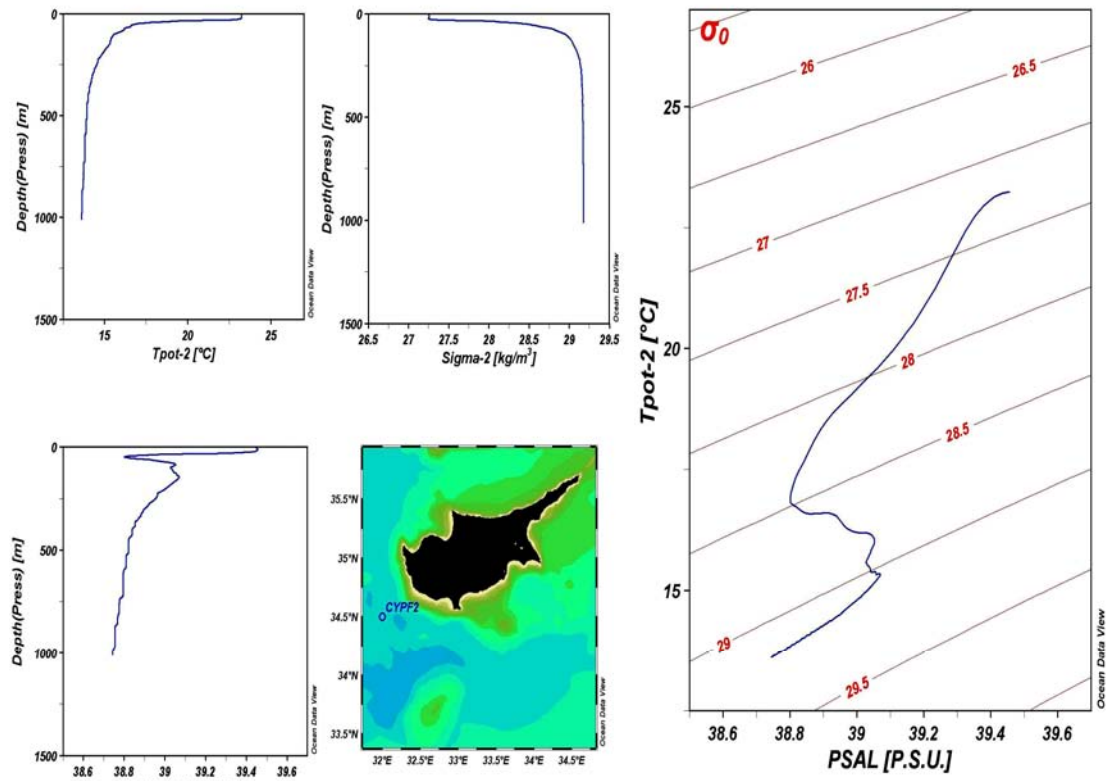
Σταθμός CYPF2, Τέλος Καλοκαιριού του 1995 (Δυναμική θερμοκρασία, αλατότητα, δυναμική πυκνότητα και διάγραμμα T-S).
