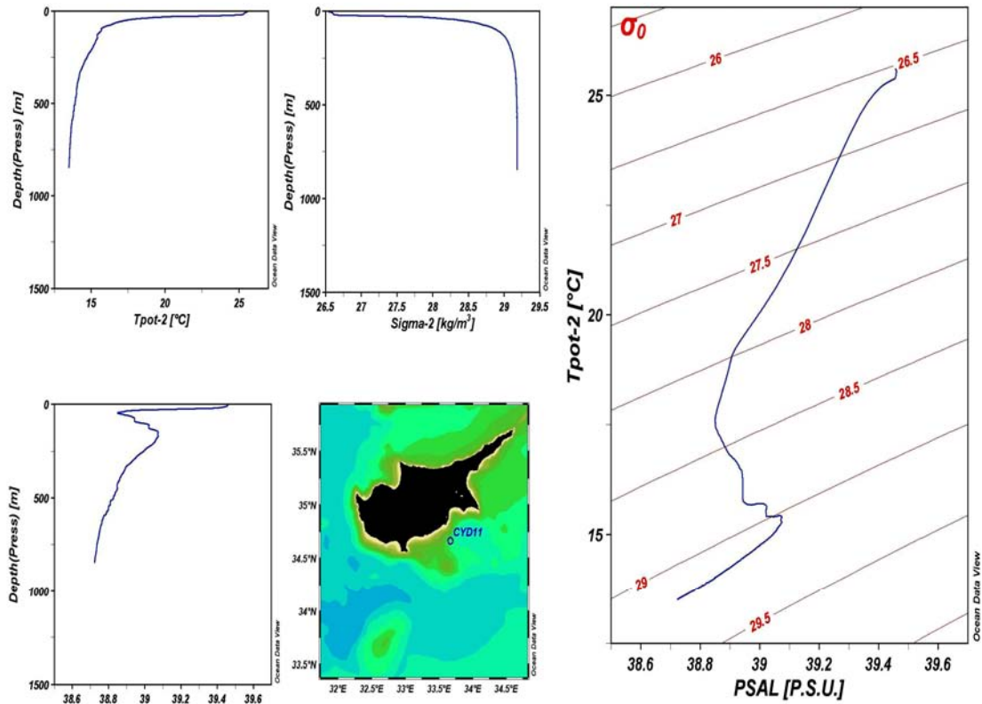
PSAL [P.S.U.] Σταθμός CYD11, Τέλος Καλοκαιριού του 1995 (Δυναμική θερμοκρασία, αλατότητα, δυναμική πυκνότητα και διάγραμμα T-S).
