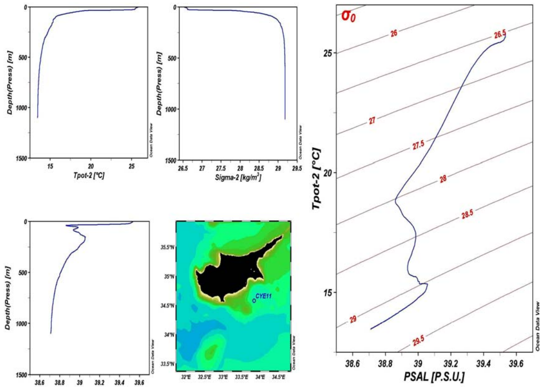
PSAL [P.S.U.] Σταθμός CYE11, Τέλος Καλοκαιριού του 1995 (Δυναμική θερμοκρασία, αλατότητα, δυναμική πυκνότητα και διάγραμμα T-S).
