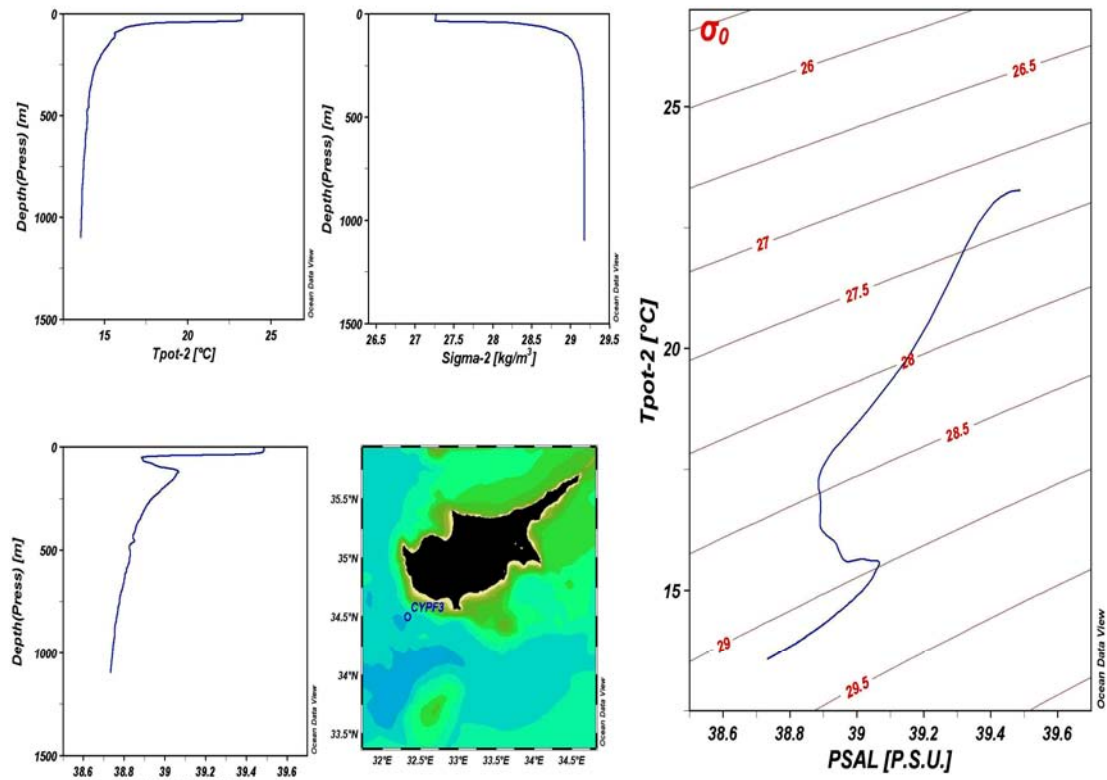
Σταθμός CYPF3, Τέλος Καλοκαιριού του 1995 (Δυναμική θερμοκρασία, αλατότητα, δυναμική πυκνότητα και διάγραμμα T-S).
