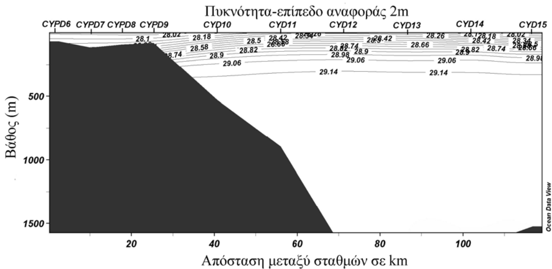
Εικόνα 3.1.2.68: Εγκάρσια τομή της πυκνότητας – A12
