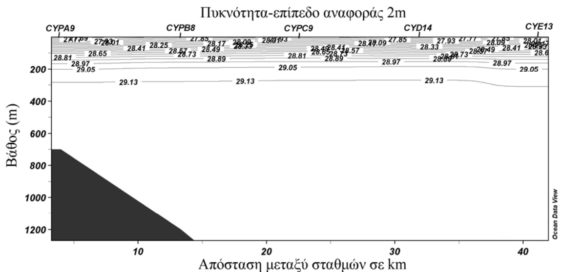
Εικόνα 3.1.2.44: Εγκάρσια τομή της πυκνότητα – Α8
