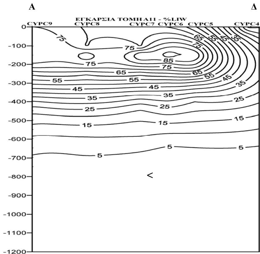
Εικόνα 3.4.2.23: Ποσοστό συμμετοχής του LIW κατά μήκος της τομής Α11.
