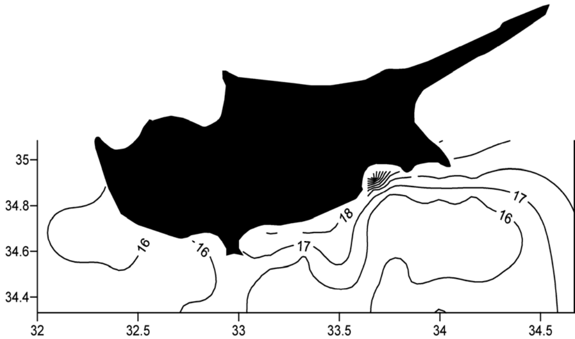
Εικόνα 3.4.3.1: Οριζόντια κατανομή της θερμοκρασίας του πυρήνα του MAW.
