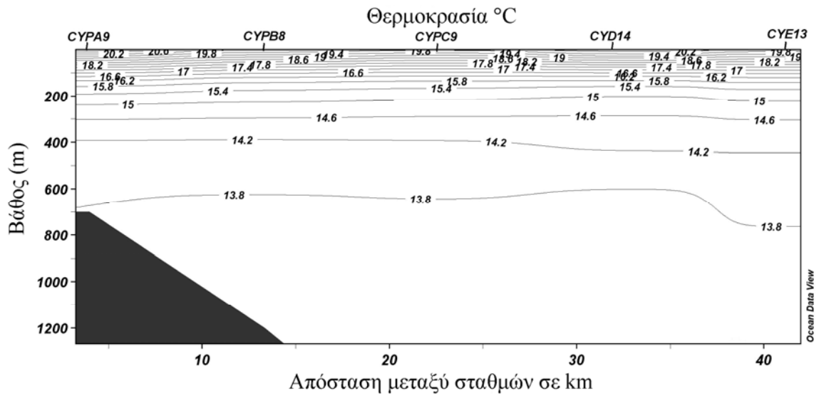
Εικόνα 3.1.2.42: Εγκάρσια τομή θερμοκρασίας-Α8
