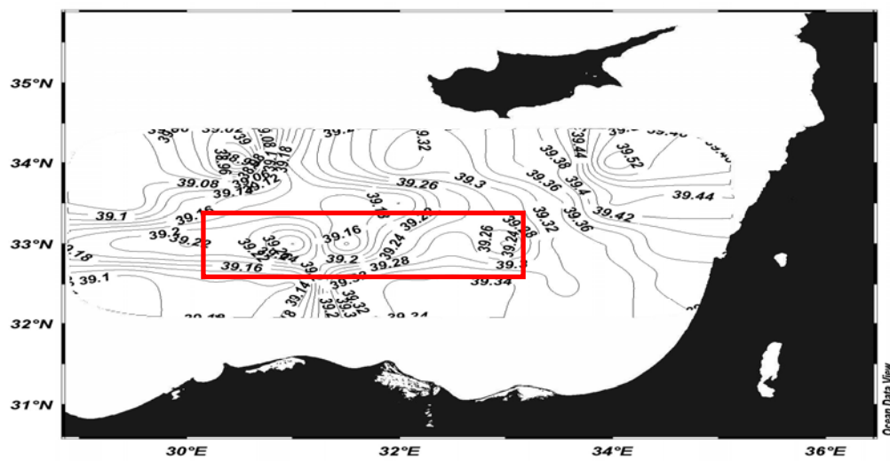
Εικόνα 3.2.1.2: Οριζόντια κατανομή της αλατότητας (2 m)
