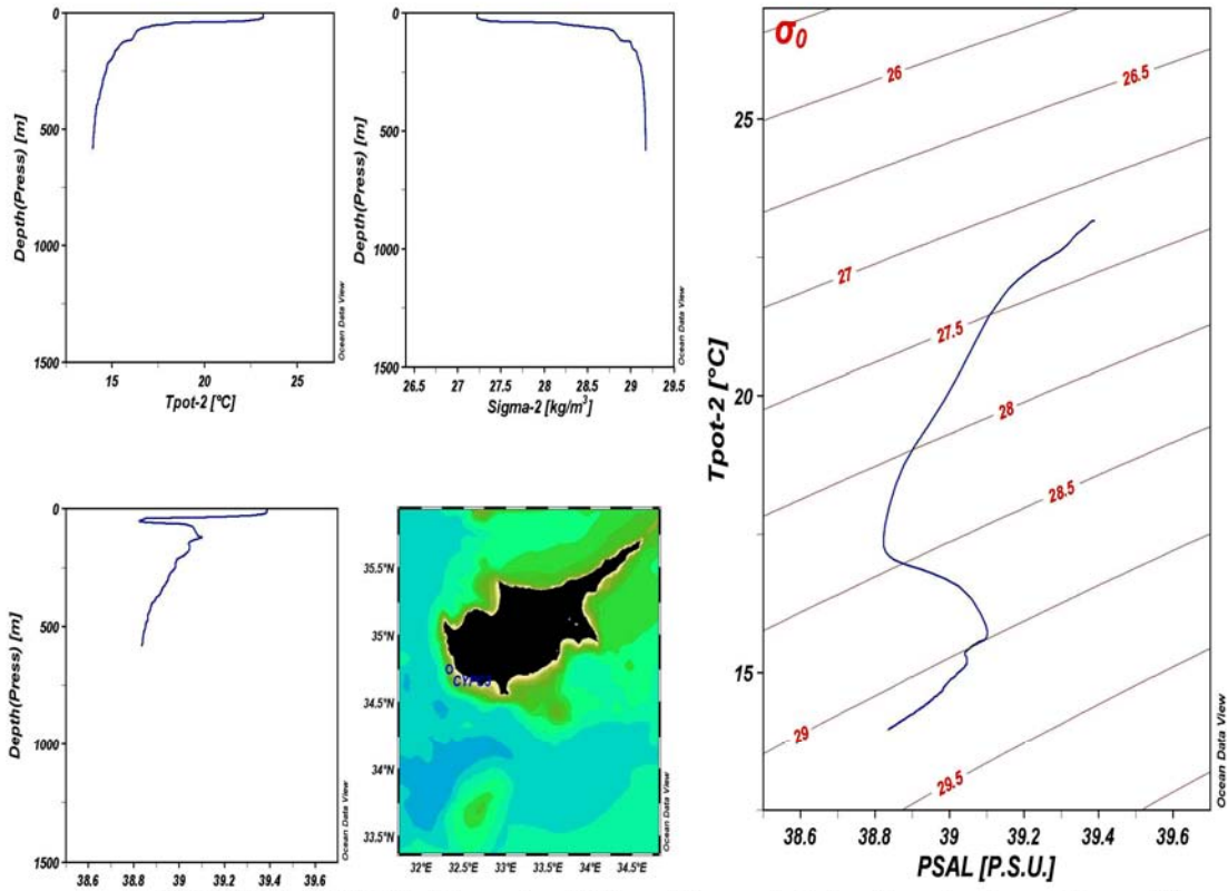
PSAL [P.S.U.] Σταθμός CYPC3, Τέλος Καλοκαιριού του 1995 (Δυναμική θερμοκρασία, αλατότητα, δυναμική πυκνότητα και διάγραμμα T-S).
