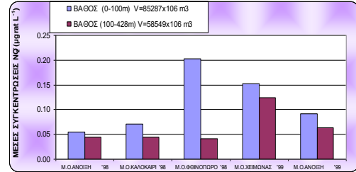
Εικόνα 3.34: Εποχιακή μεταβολή μέσης συγκέντρωσης NO 2 -
