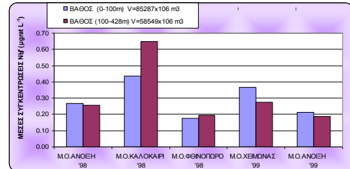
Εικόνα 3.36: Εποχιακή μεταβολή μέσης συγκέντρωσης NH 4 +
