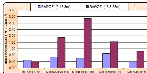
Εικόνα 3.12: Εποχιακή μεταβολή μέσης συγκεντρώσεως \text{NH}_4^+
