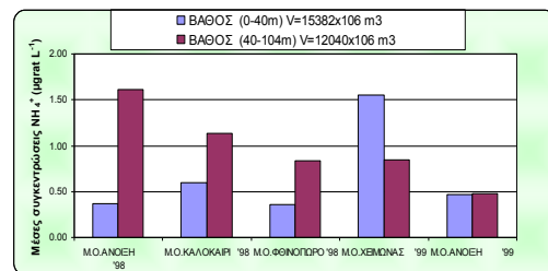
Εικόνα 3.24: Εποχιακή μεταβολή μέσης συγκέντρωσης NH 4 +
