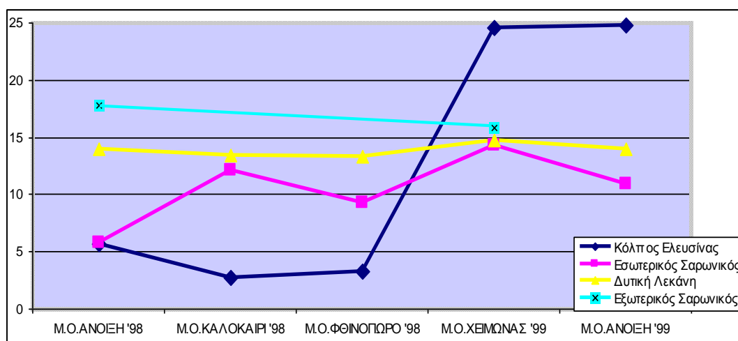
Εικόνα 3.41: Εποχιακή μεταβολή του λόγου ΣΝ/ΣΡ για τις επιμέρους περιοχές του Σαρωνικού κόλπου την περίοδο 05/1998 – 05/1999
