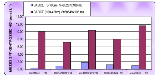
Εικόνα 3.35: Εποχιακή μεταβολή μέσης συγκέντρωσης NO 3 -
