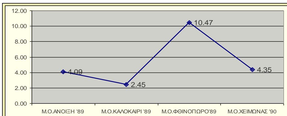
Εικόνα 2.21: Εποχιακή μεταβολή του Λόγου ΣΝ/ΣΡ για τον κόλπο Ελευσίνας (περίοδος 04/1989 – 03/1990)
