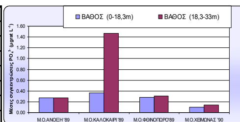
Εικόνα 3.2: Εποχιακή μεταβολή μέσης συγκεντρώσεως PO_4^{3-}
