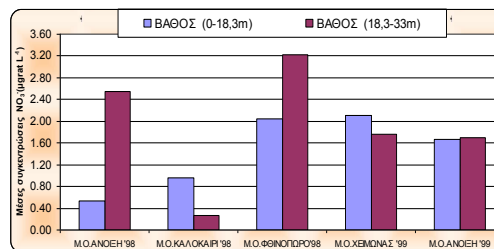
Εικόνα 3.11: Εποχιακή μεταβολή μέσης συγκεντρώσεως \text{NO}_3^-
