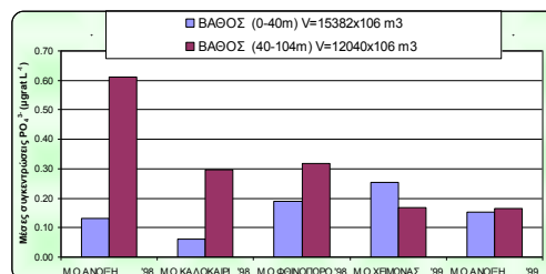
Εικόνα 3.20: Εποχιακή μεταβολή μέσης συγκέντρωσης \text{PO}_4^{3-}
