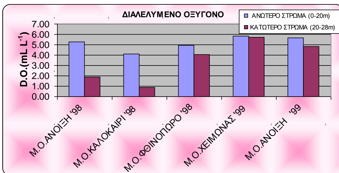
Εικόνα Π.2: Γράφημα εποχιακών μεταβολών συγκέντρωσης διαλελυμένου οξυγόνου (05/1998-05/1999)
