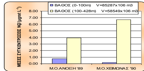
Εικόνα 3.29: Εποχιακή μεταβολή μέσης συγκέντρωσης NO 3 -
