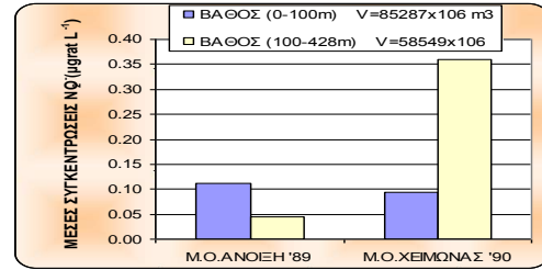
Εικόνα 3.28: Εποχιακή μεταβολή μέσης συγκέντρωσης NO 2 -
