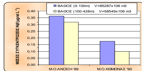
Εικόνα 3.30: Εποχιακή μεταβολή μέσης συγκέντρωσης NH 4 +
