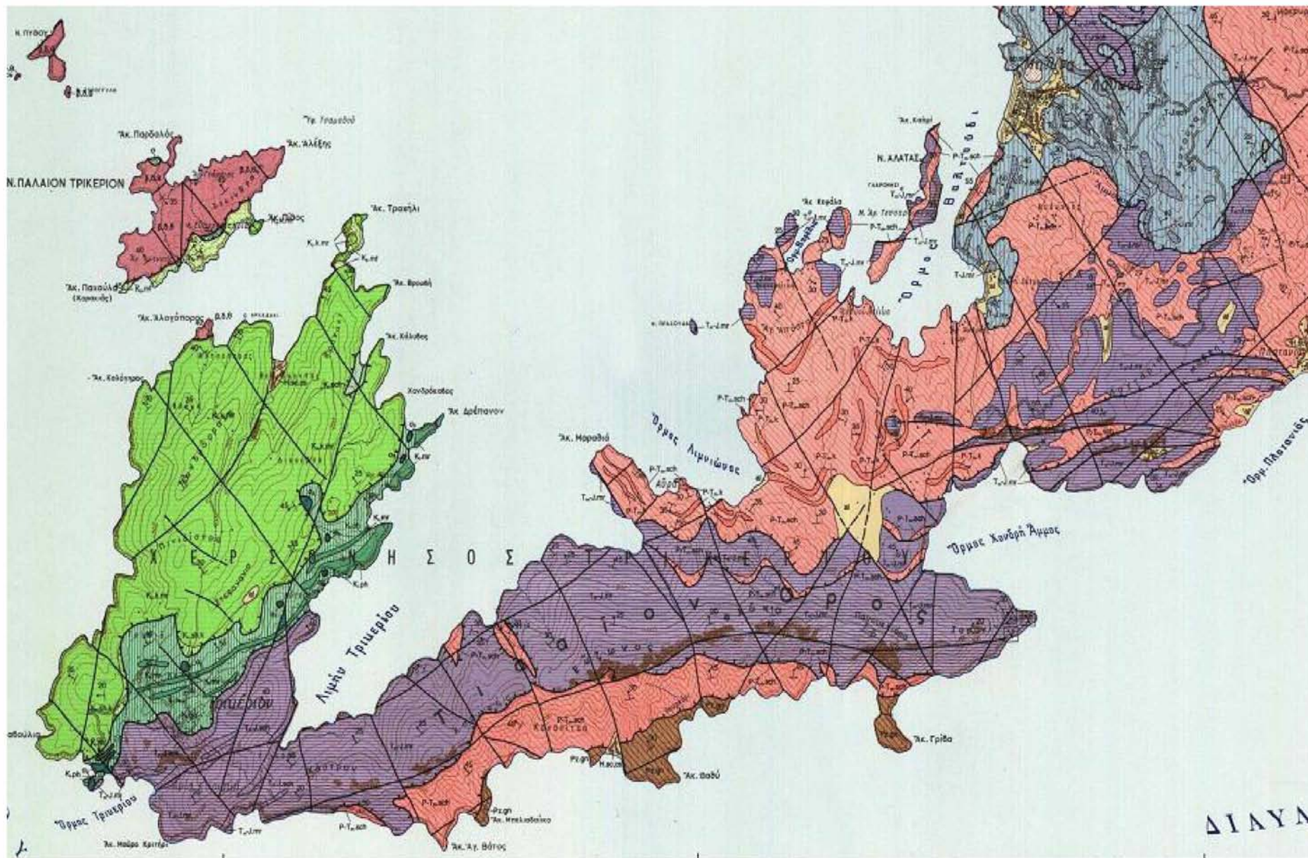
Εικόνα 10. Γεωλογικός Χάρτης Περιοχής Τρικερίου
