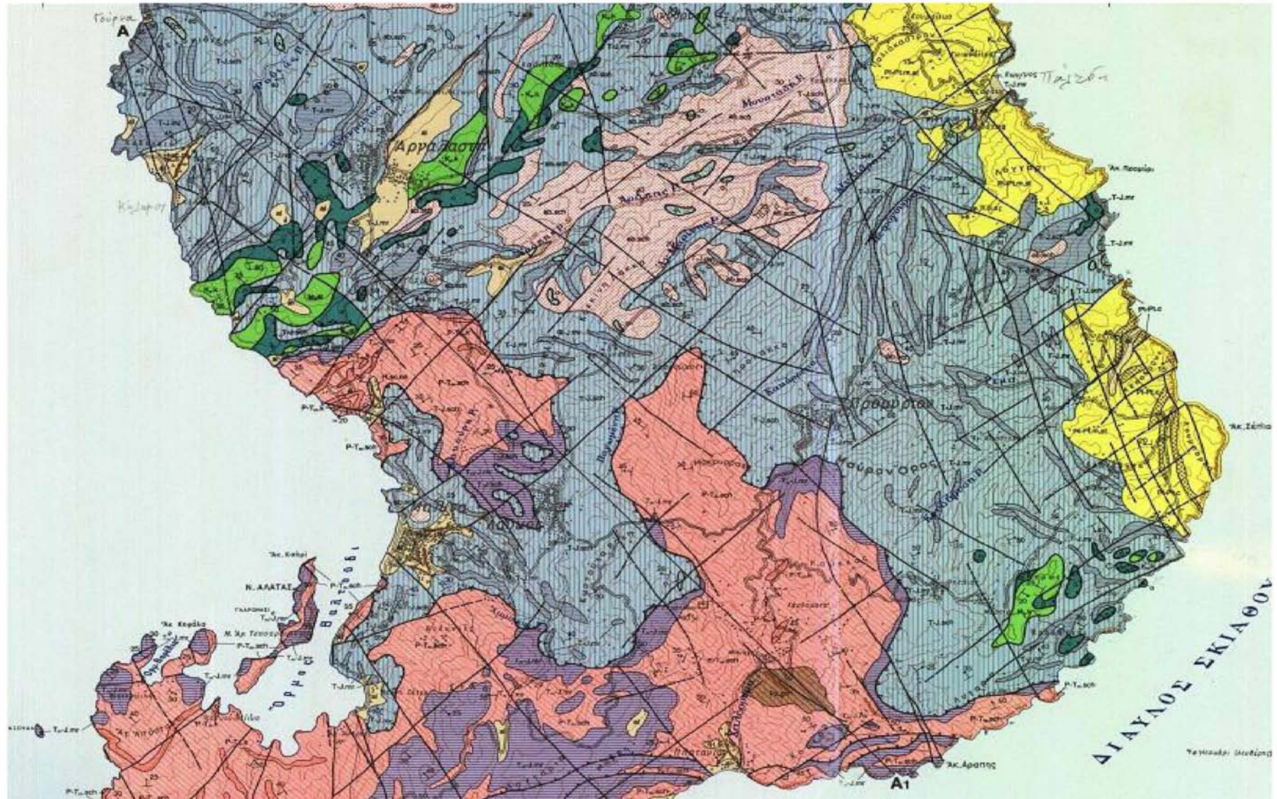
Εικόνα 9. Γεωλογικός Χάρτης Περιοχής Αργολαστικής
