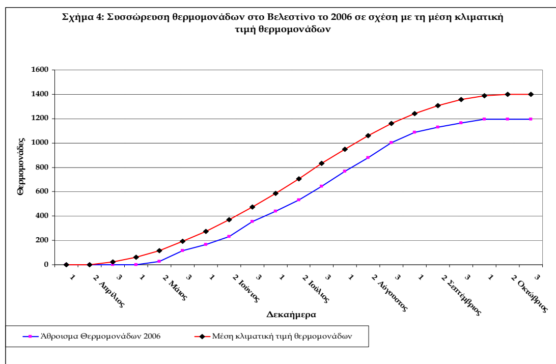
Σχήμα 4. Συσώρευση θερμομονάδων στο Βελεστίνο το 2006 σε σχέση με τη μέση κλιματική τιμή θερμομονάδων (βασική θερμοκρασία 15,6° C).
