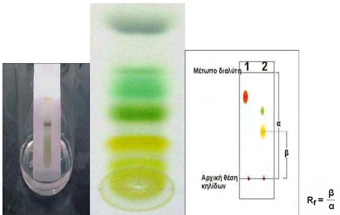
Εικόνα 3.1 Παράδειγμα χρωματογραφίας λεπτής στιβάδας
