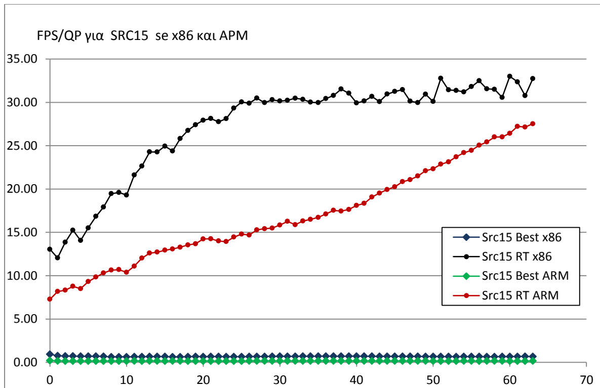
Σχήμα 22.4.15: FPS/QP για src15 με VP8
