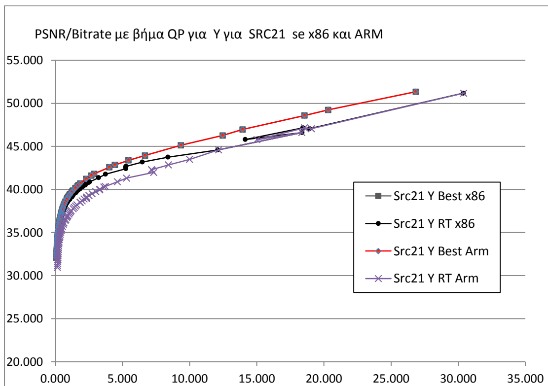
Σχήμα 22.1.20: Λόγος PSNR/Bitrate με βήμα QP για τη συνιστώσα Y για SRC21 σε x86 και ARM
