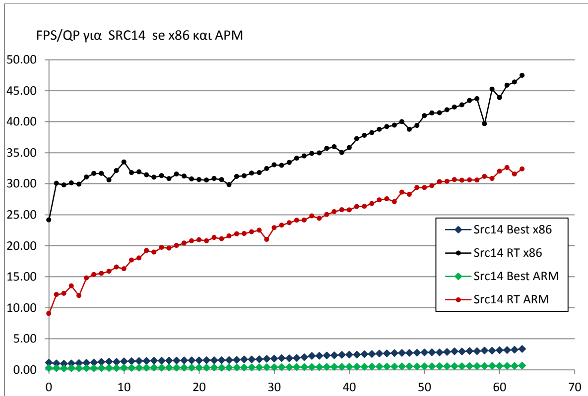
Σχήμα 22.4.14: FPS/QP για src14 με VP8
