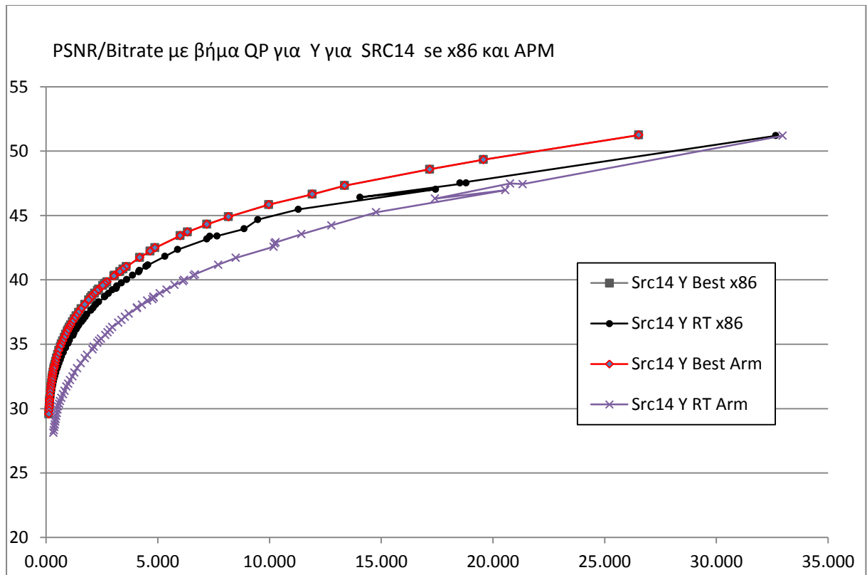
Σχήμα 22.1.14: Λόγος PSNR/Bitrate με βήμα QP για τη συνιστώσα Y για SRC14 σε x86 και APM
