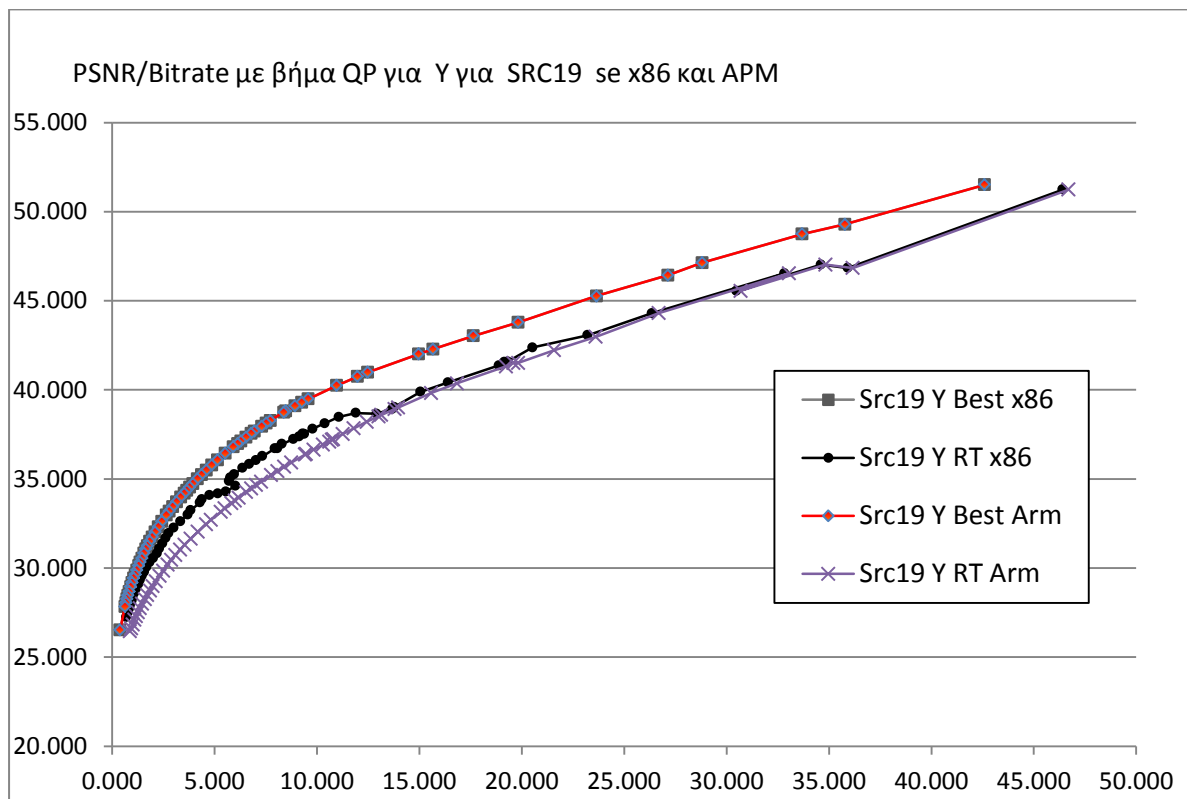
Σχήμα 22.1.19: Λόγος PSNR/BiRate με βήμα QP για τη συνιστώσα Y για SRC19 σε x86 και APM
