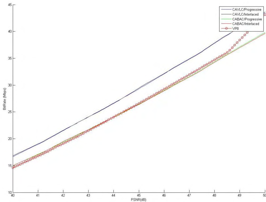
Σχήμα 22.8.3: Bitrate/PSNR για Y για SRC15 για VP8 και H.264 για εύρος 40 db έως 50 db
