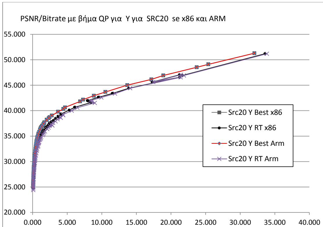
Σχήμα 22.1.20: Λόγος PSNR/Bitrate με βήμα QP για τη συνιστώσα Y για SRC20 σε x86 και ARM
