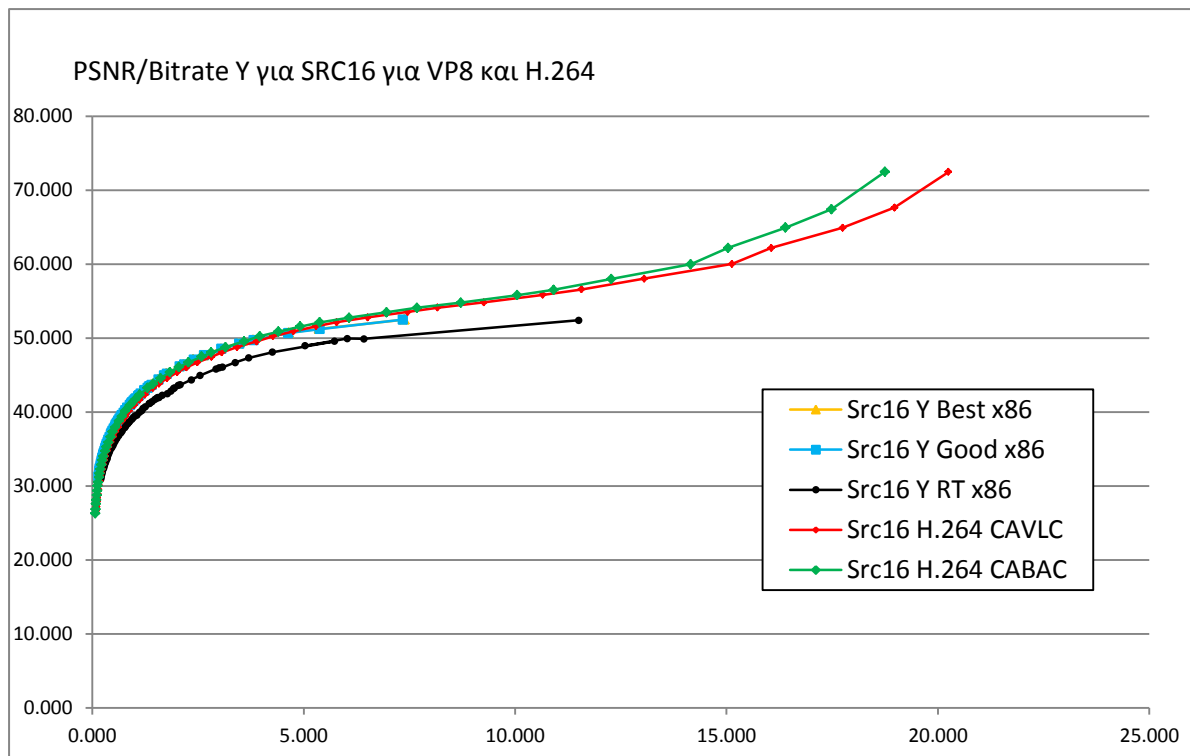
Σχήμα 22.7.16: PSNR/Bitrate Y για SRC16 για VP8 και H.264
