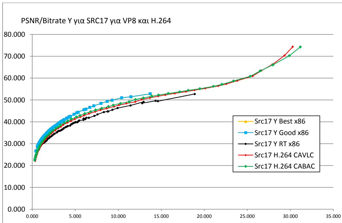
Σχήμα 22.7.17: PSNR/Bitrate Y για SRC17 για VP8 και H.264
