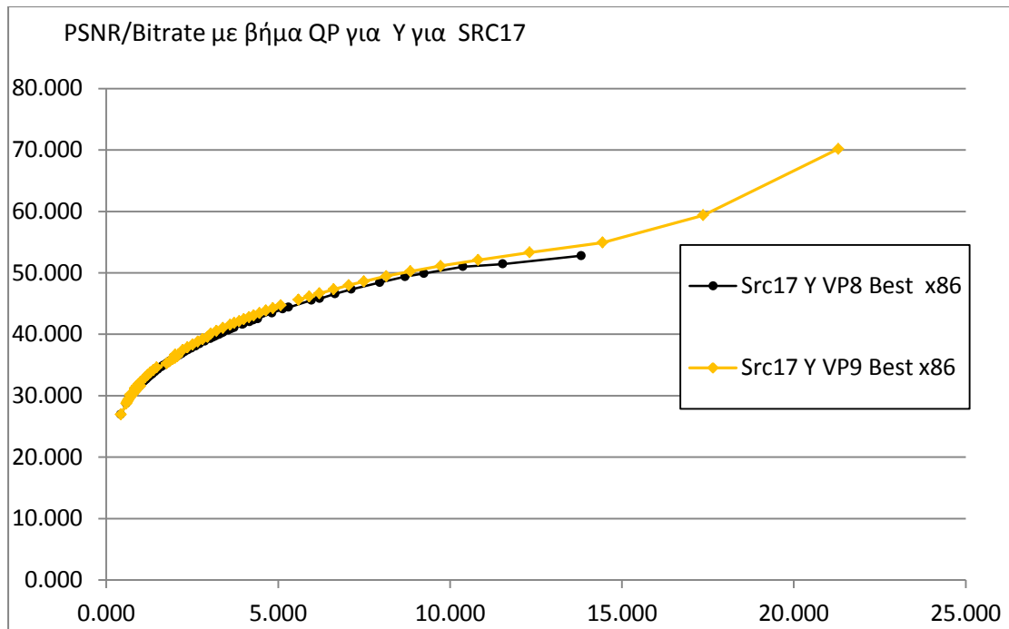
Σχήμα 37: Αποδοτικότητα VP9 σε σχέση με τον VP8 για src17.
