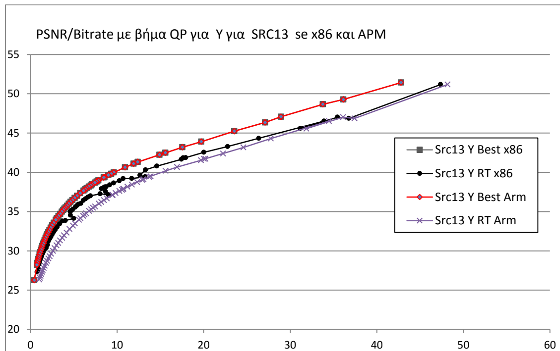
Σχήμα 22.1.13: Λόγος PSNR/Bitrate με βήμα QP για τη συνιστώσα Y για SRC13 σε x86 και ARM
