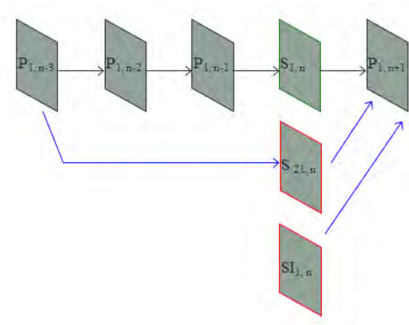
Σχήμα 12: Παράδειγμα χρήσης SI-frames για Error Recovery/Resiliency
