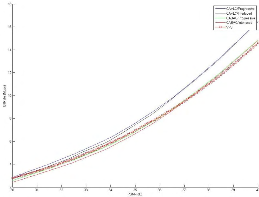
Σχήμα 22.8.2: Bitrate/PSNR για Y για SRC15 για VP8 και H.264 για εύρος 30 db έως 40 db
