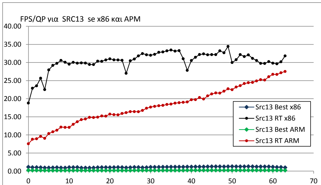
Σχήμα 22.4.13: FPS/QP για src13 με VP8
