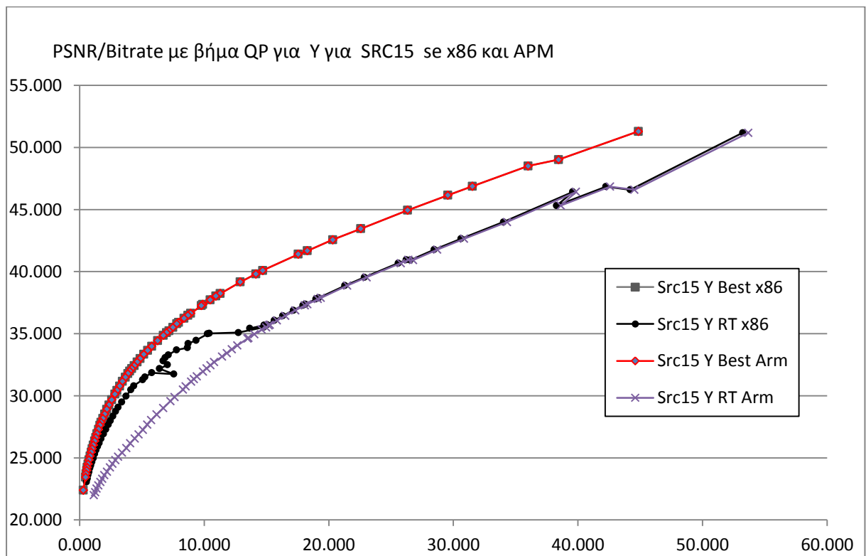
Σχήμα 22.1.15: Λόγος PSNR/Bitrate με βήμα QP για τη συνιστώσα Y για SRC15 σε x86 και APM
