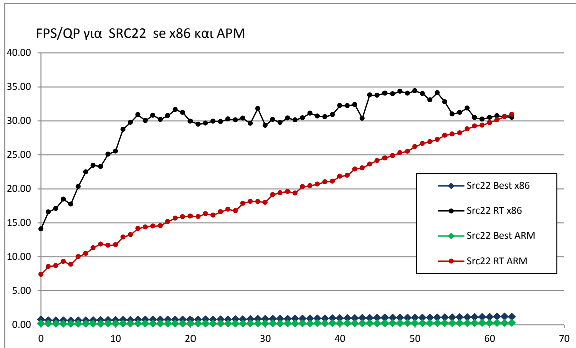
Σχήμα 22.4.22: FPS/QP για src22 με VP8
