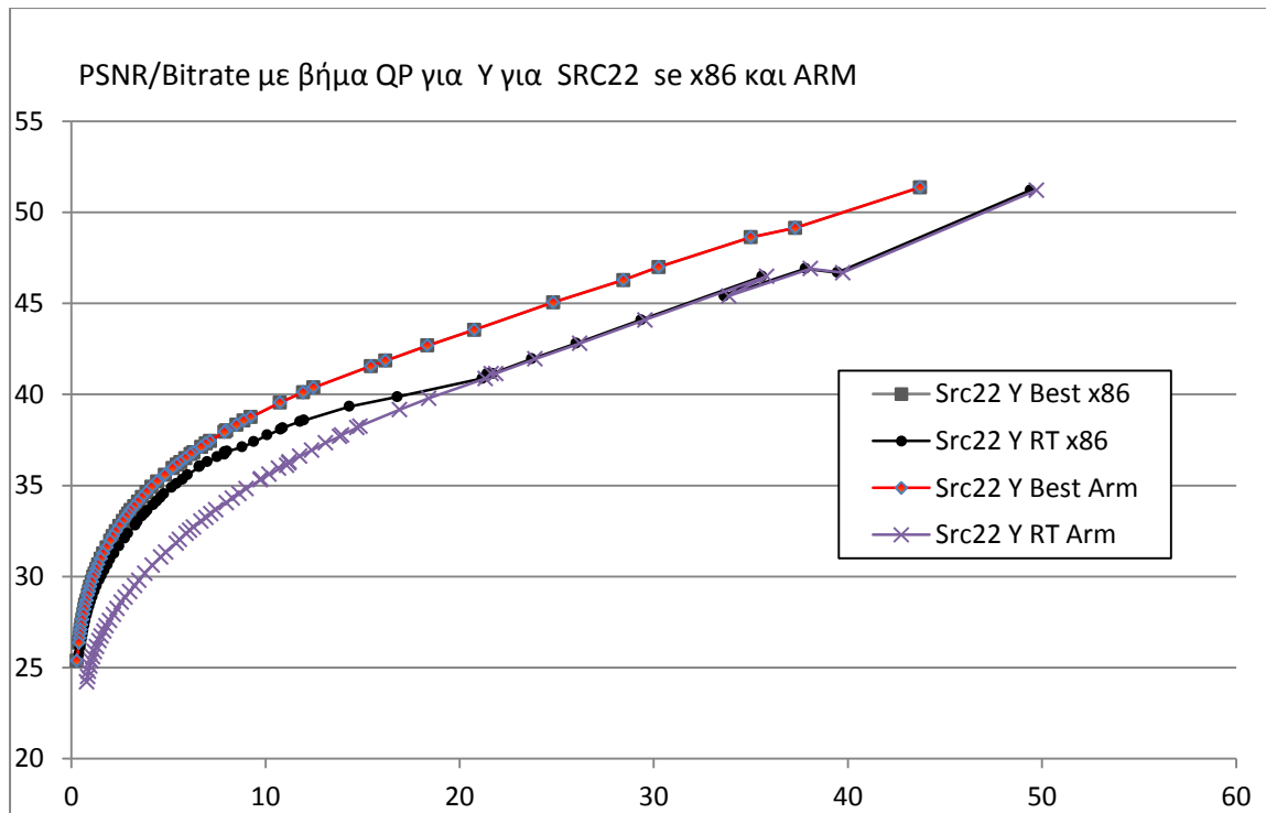
Σχήμα 22.1.20: Λόγος PSNR/Bitratio με βήμα QP για τη συνιστώσα Y για SRC22 σε x86 και ARM
