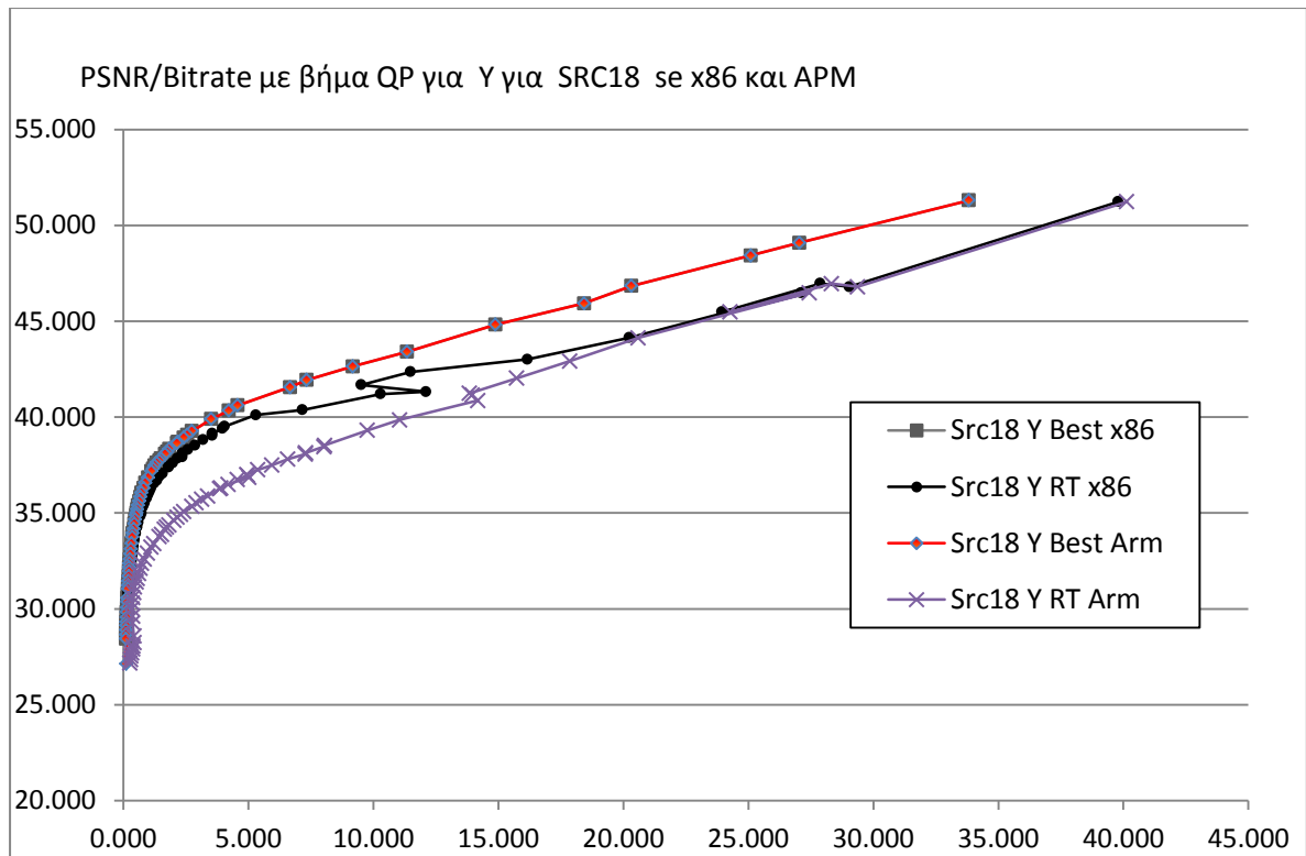
Σχήμα 22.1.18: Λόγος PSNR/BiRate με βήμα QP για τη συνιστώσα Y για SRC18 σε x86 και APM
